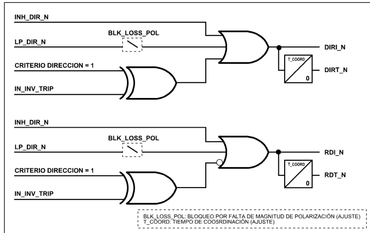
Figura 3.2.9: Diagrama de operación de la unidad direccional de neutro.
