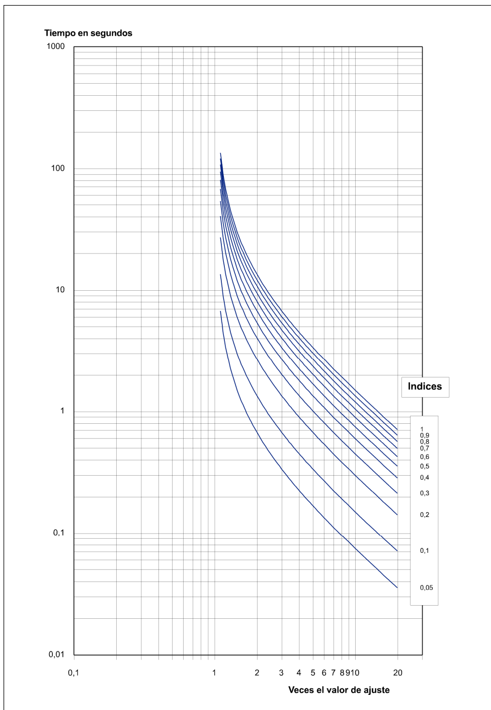
Figura 3.1.5: Característica MUY INVERSA (IEC)
