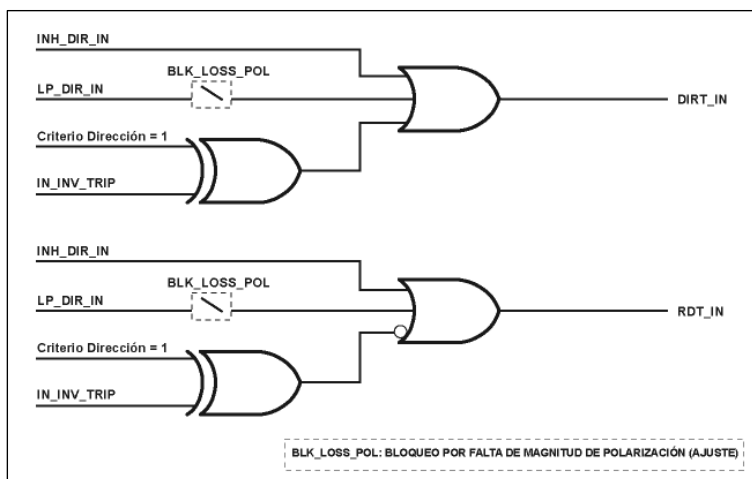
Figura 3.2.2: Diagrama de operación de la unidad direccional de fases.
