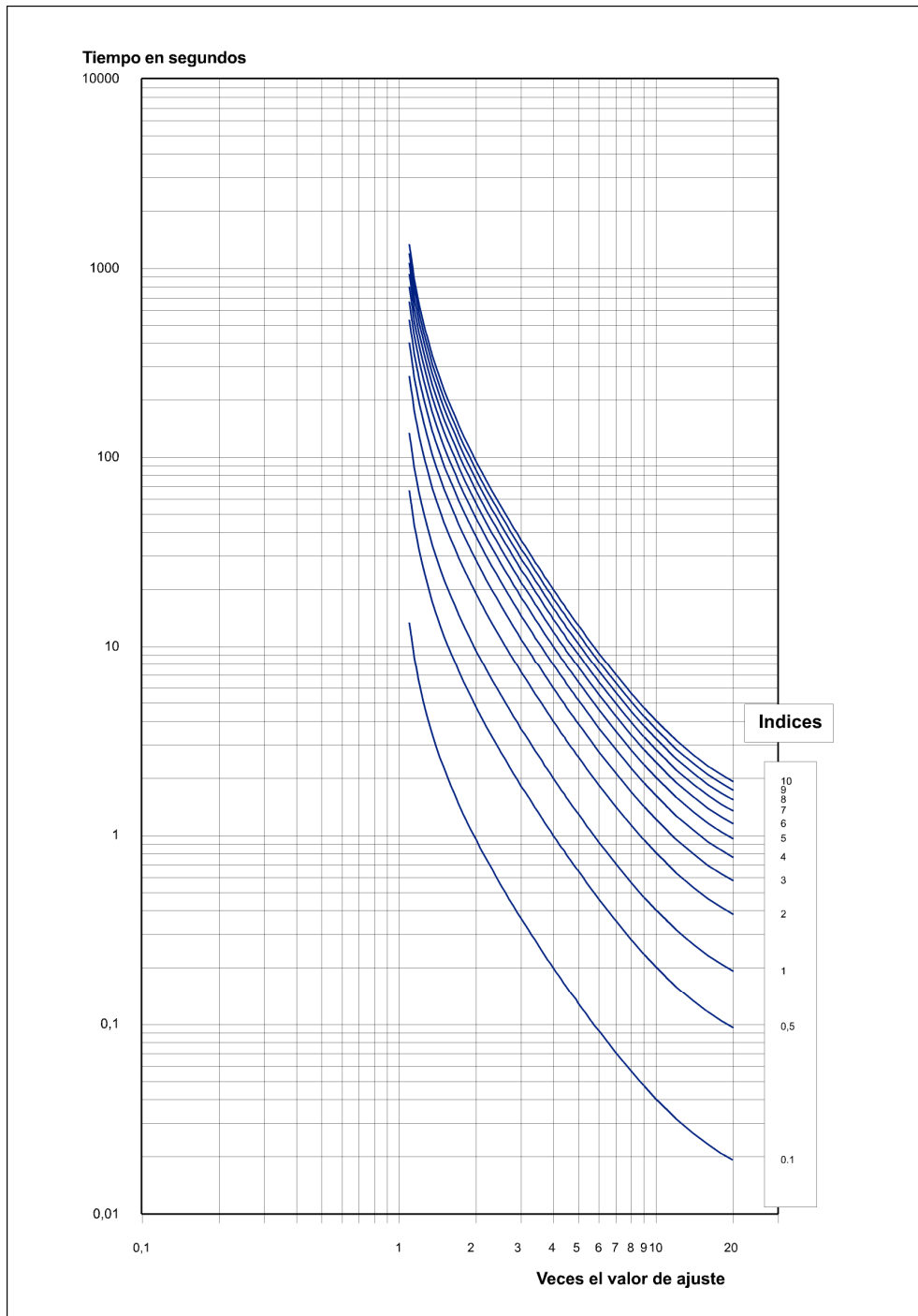
Figura 3.1.11: Característica EXTREMADAMENTE INVERSA (IEEE)
