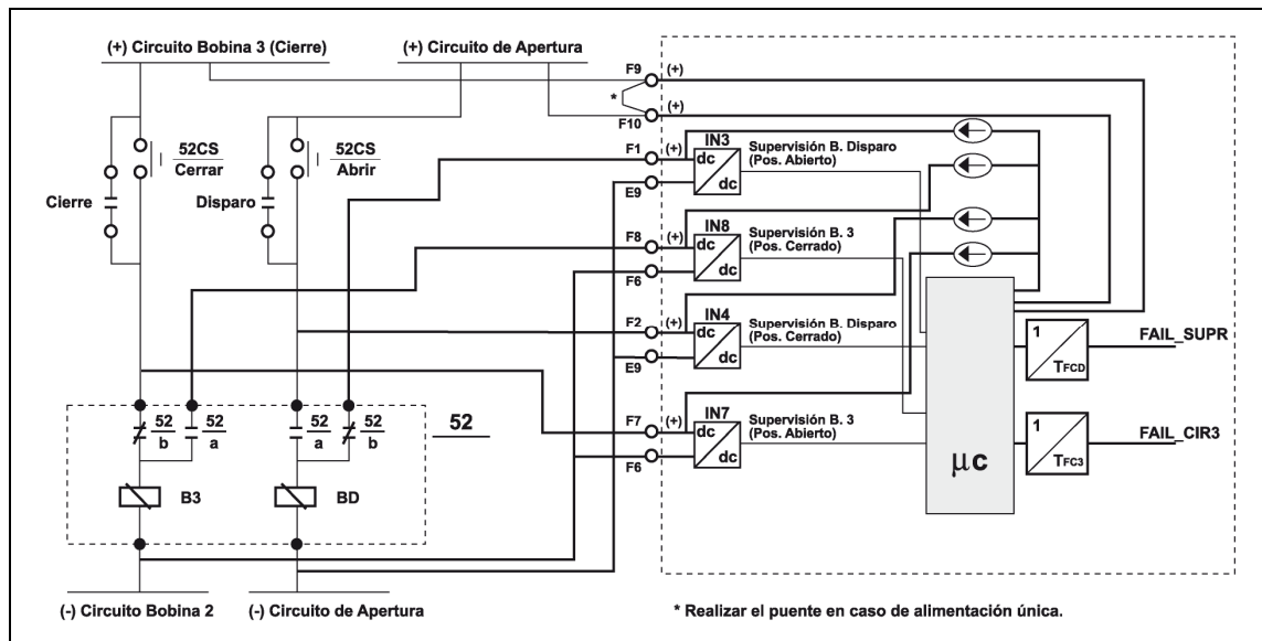
Figura 3.28.1: Diagrama de bloques y aplicación de las funciones de supervisión de circuitos de maniobra (I)
