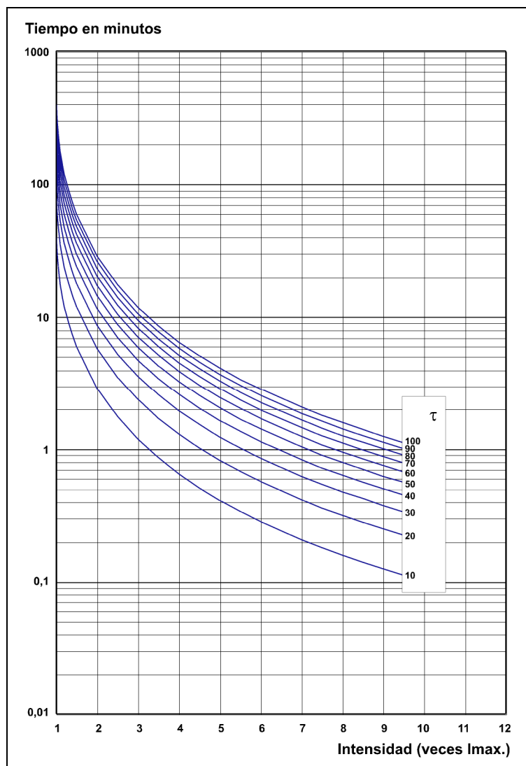
Figura 3.13.2: Curvas características del tiempo de operación de la unidad térmica
