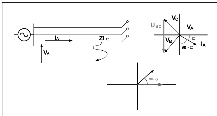
Figura 3.2.3: Gráficas para el ejemplo de aplicación.
