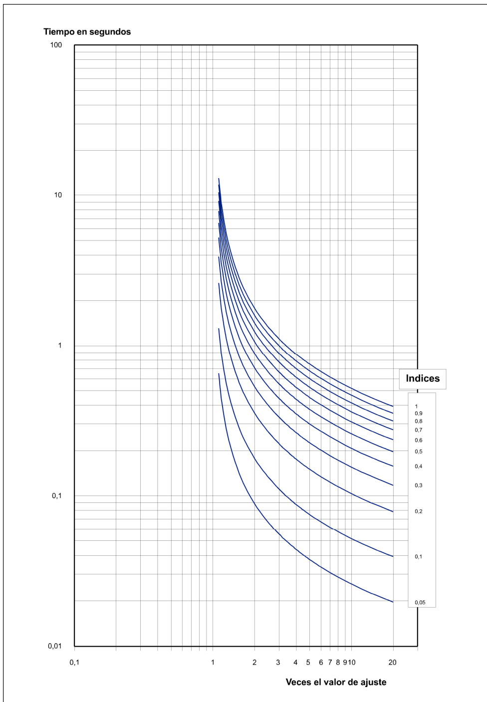
Figura 3.1.8: Característica TIEMPO-CORTO INVERSA (IEC)
