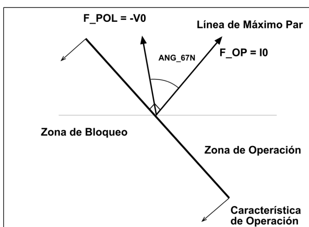
Figura 3.2.4: Diagrama vectorial de la unidad direccional de neutro (polarización por tensión).
