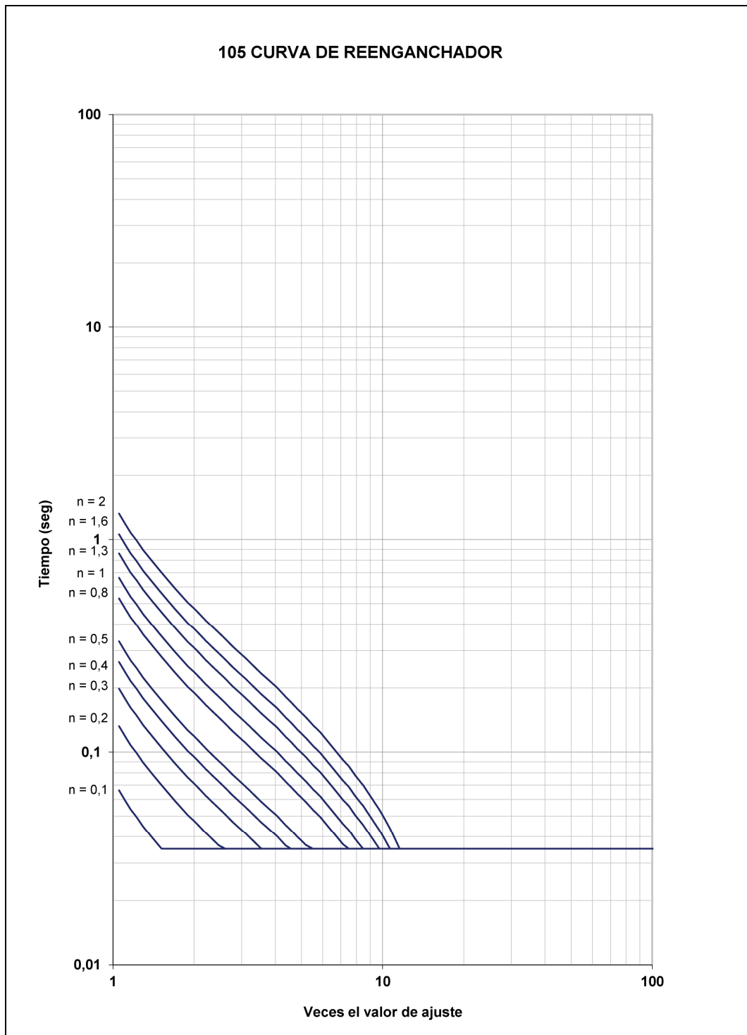
Figura 3.1.19: 105 curva de reenganchador
