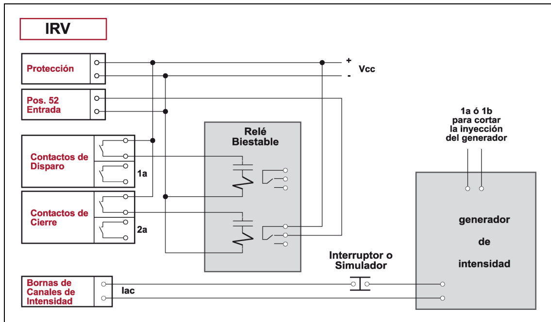
Figura 3.23.6: Esquema de conexión para el ensayo del reenganchador.
