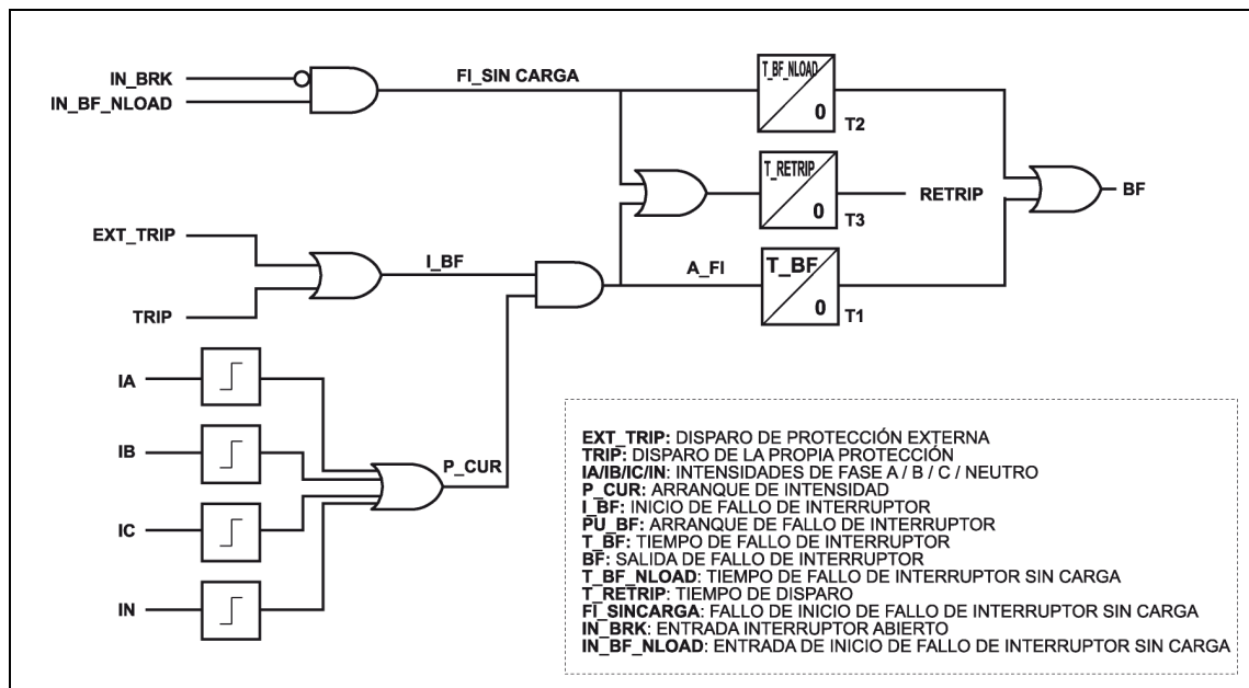
Figura 3.8.2: Diagrama de bloques de la unidad de fallo de interruptor (IRV-J)
