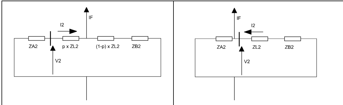
Figura 3.2.12: Red de secuencia inversa para falta hacia adelante.
