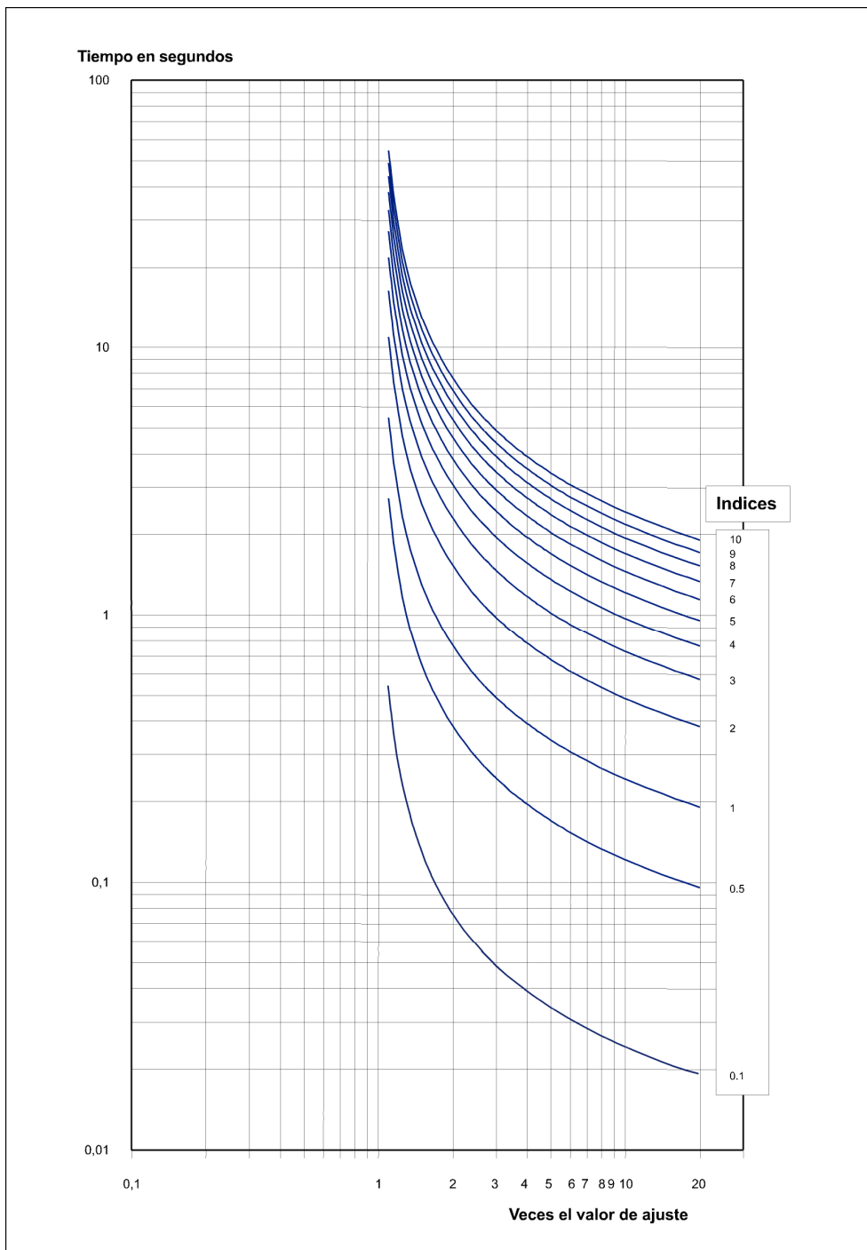
Figura 3.1.12: Característica MODERADAMENTE INVERSA (U.S.)
