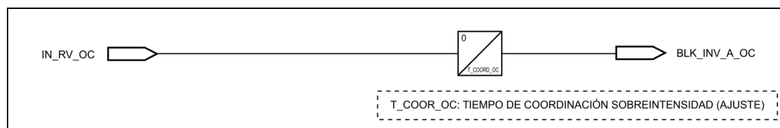
Figura 3.3.8: Diagrama de bloques de la lógica de bloqueo transitorio por inversión de intensidad
