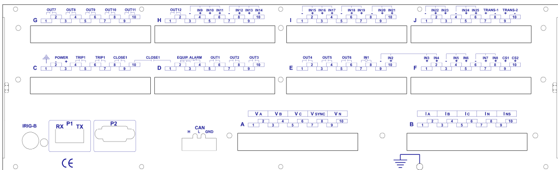
Figura 2.3.4: Trasera de un 8IRV de 3U de altura
