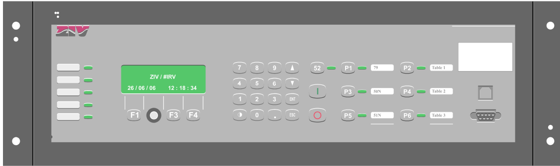
Figura 2.3.16: Frente de un 8IRV de 3U de altura con tapa de protección
