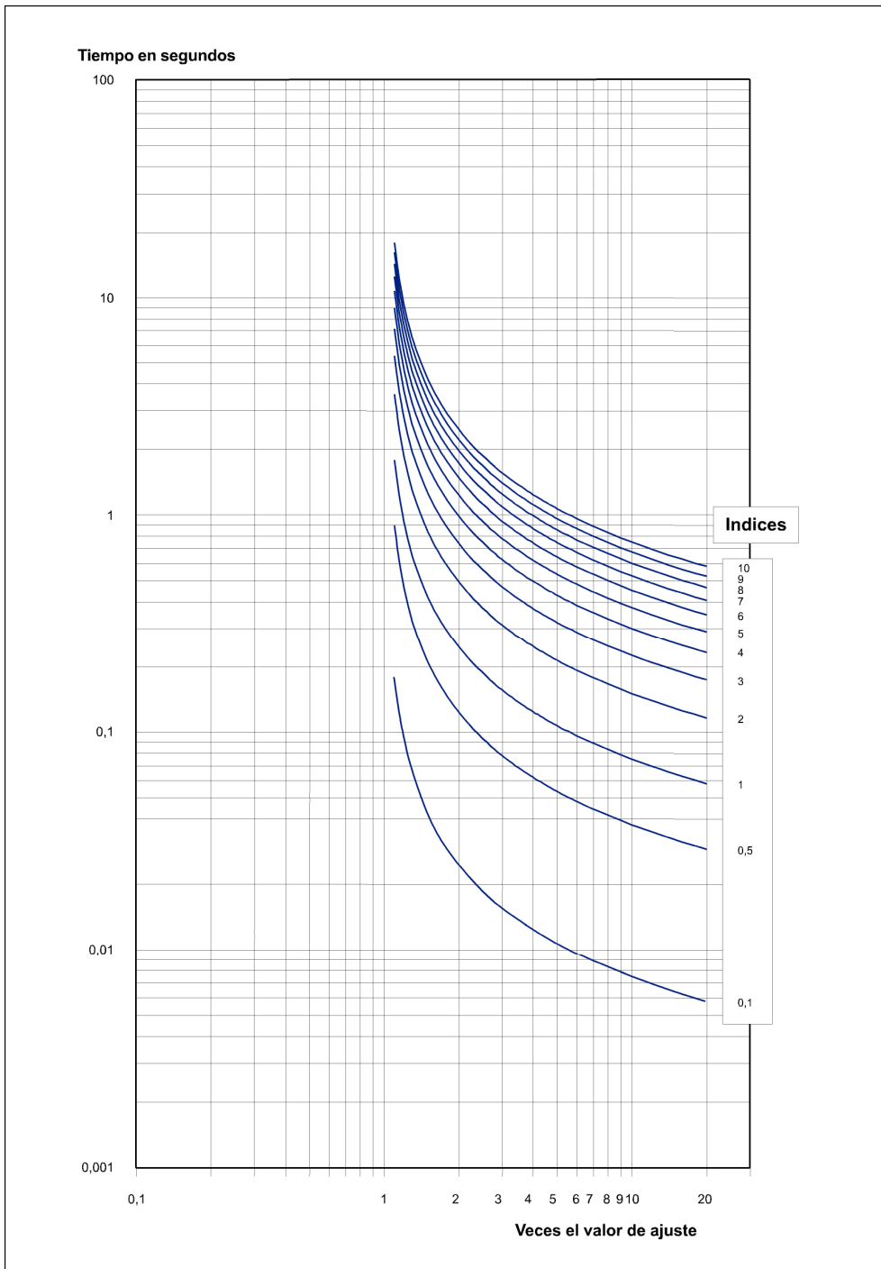
Figura 3.1.16: Característica INVERSA DE TIEMPO CORTO (U.S.)
