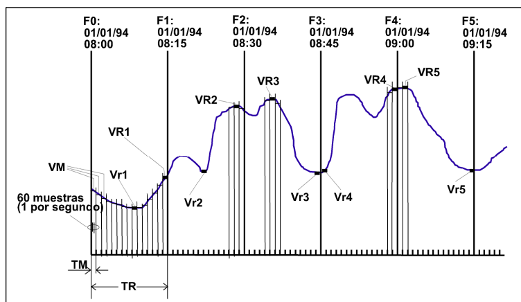
Figura 3.35.1: Diagrama explicativo del registro histórico
