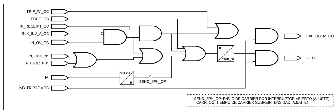
Figura 3.3.4: Diagrama de bloques del esquema de desbloqueo por comparación direccional (IRV-D/G/H****Y0 e IRV-J)
