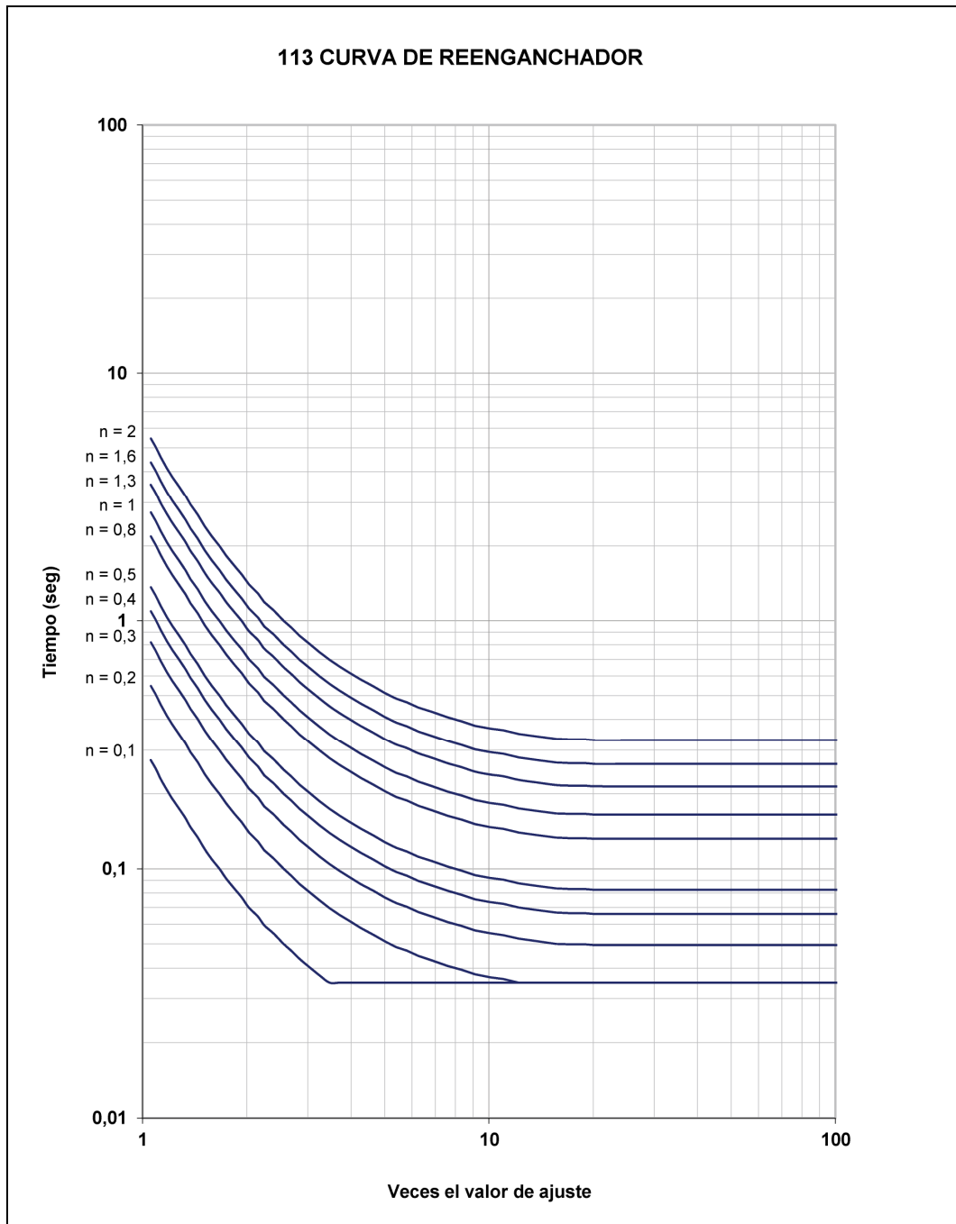
Figura 3.1.21: 113 curva de reenganchador
