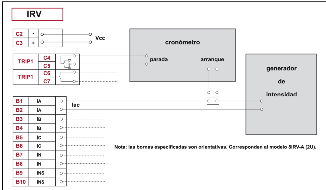
Figura 3.6.4: Esquema de conexión para el ensayo de medida de tiempos.
