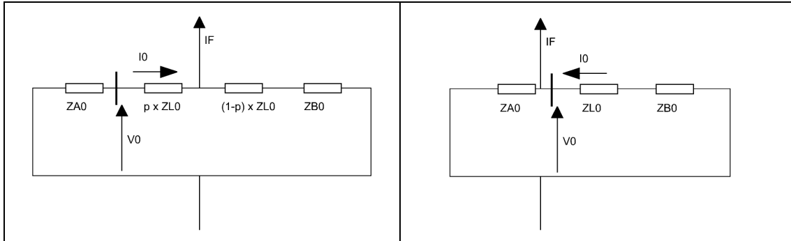
Figura 3.2.5: Red de secuencia cero para falta hacia adelante.
