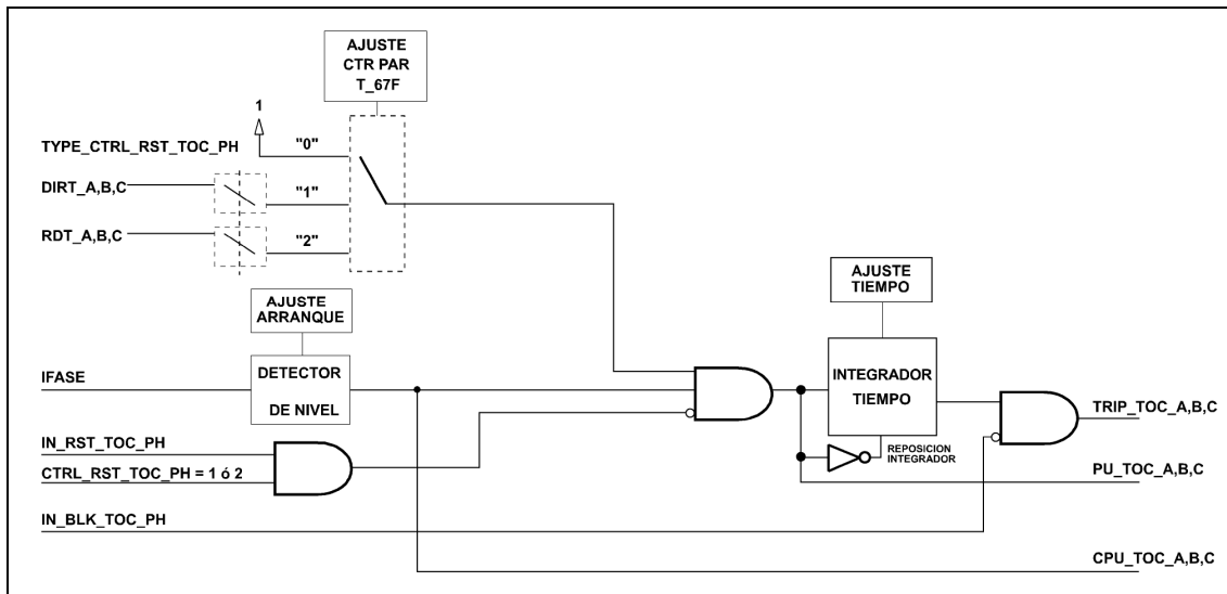
Figura 3.1.27: Diagrama de bloques de una unidad de sobrecorriente temporizada de fases
