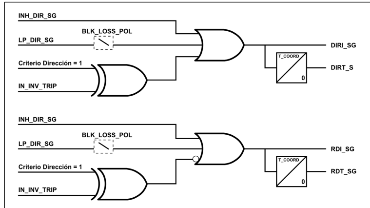
Figura 3.2.10: Diagrama de operación de la unidad direccional de neutro sensible.
