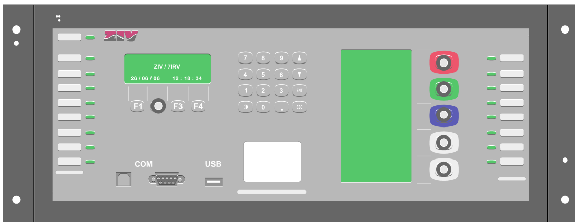
Figura 2.3.17: Frente de un 7IRV de 4U de altura con tapa de protección
