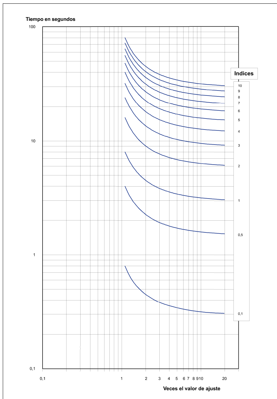
Figura 3.1.17: Característica RI INVERSA
