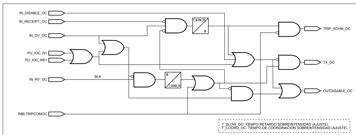
Figura 3.3.5: Diagrama de bloques del esquema de bloqueo por comparación direccional
