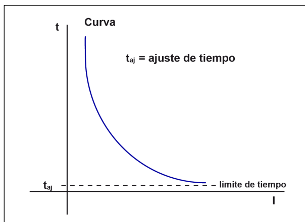
Figura 3.1.1: Curva con límite de tiempo para una unidad de sobreintensidad temporizada (ajuste de Tiempo fijo muy bajo).
