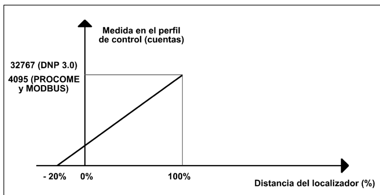
Figura 3.38.1: Escala de las medidas del localizador en el perfil de control
