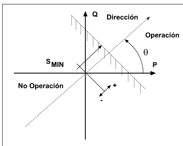
Figura 3.16.1: Operación de la unidad direccional de potencia
