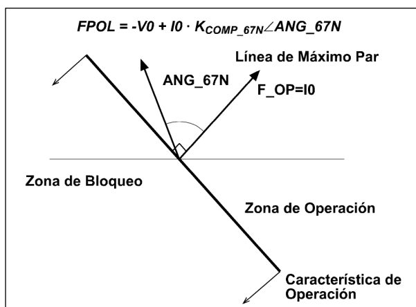
Figura 3.2.7: Diagrama vectorial de la unidad direccional de neutro en los modelos IRV-D/G/H*****Y0 e IRV-J (polarización por tensión).
