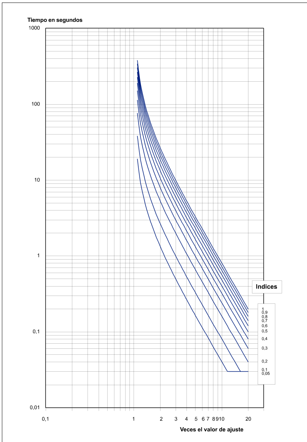
Figura 3.1.6: Característica EXTREMADAMENTE INVERSA (IEC)
