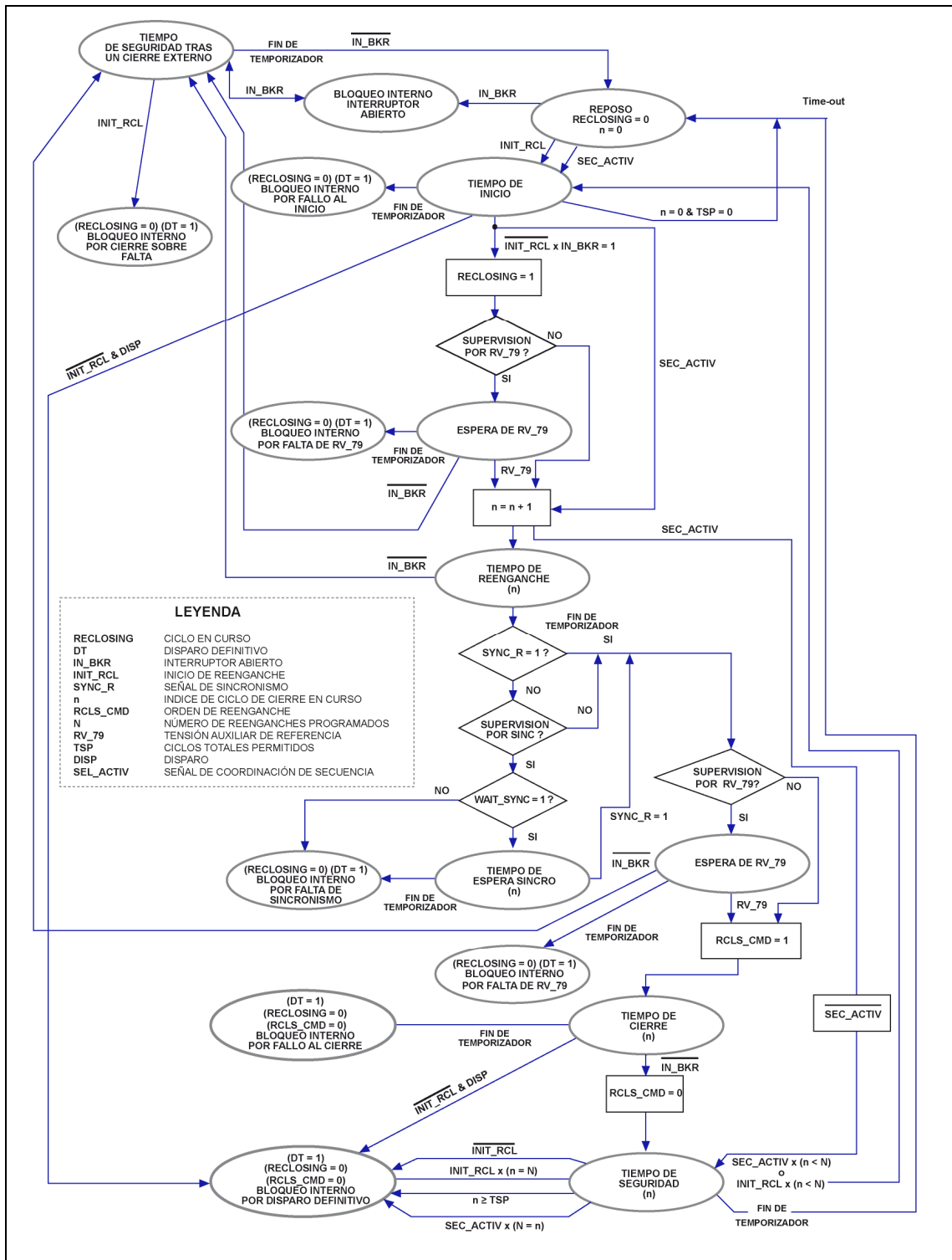
Figura 3.23.3: Diagrama de flujo del reenganchador a partir de la versión de memoria 3.20
