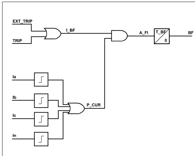
Figura 3.8.1: Diagrama de bloques de la unidad de fallo de interruptor
