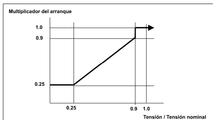
Figura 3.1.29: Unidad temporizada frenada por tensión.
