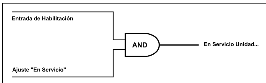
Figura 3.39.1: Lógica de habilitación de unidad
