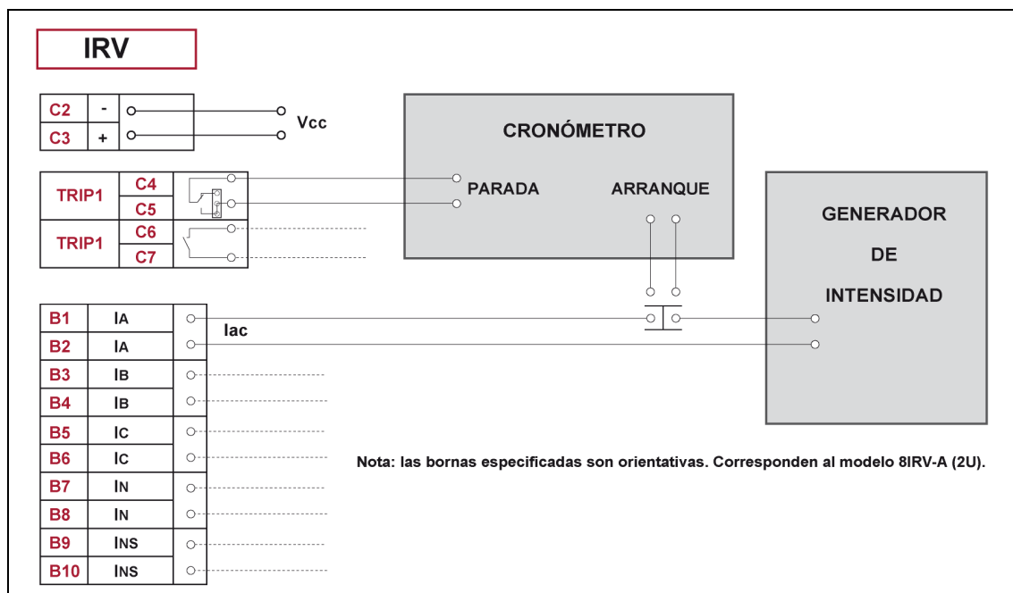
Figura 3.1.30: Esquema de conexión para el ensayo de medida de tiempos
