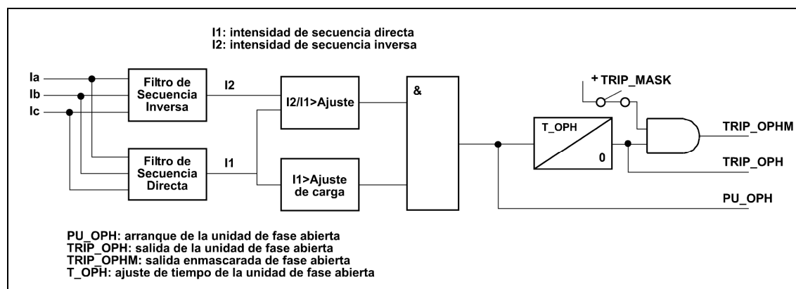
Figura 3.9.1: Diagrama de bloques de la unidad de fase abierta
