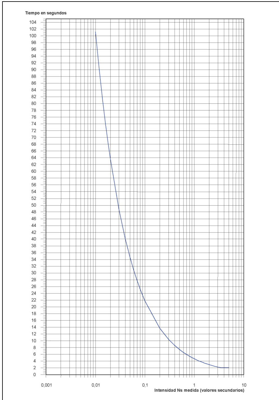
Figura 3.1.18: Característica EPATR_C (tiempo neutro sensible)
