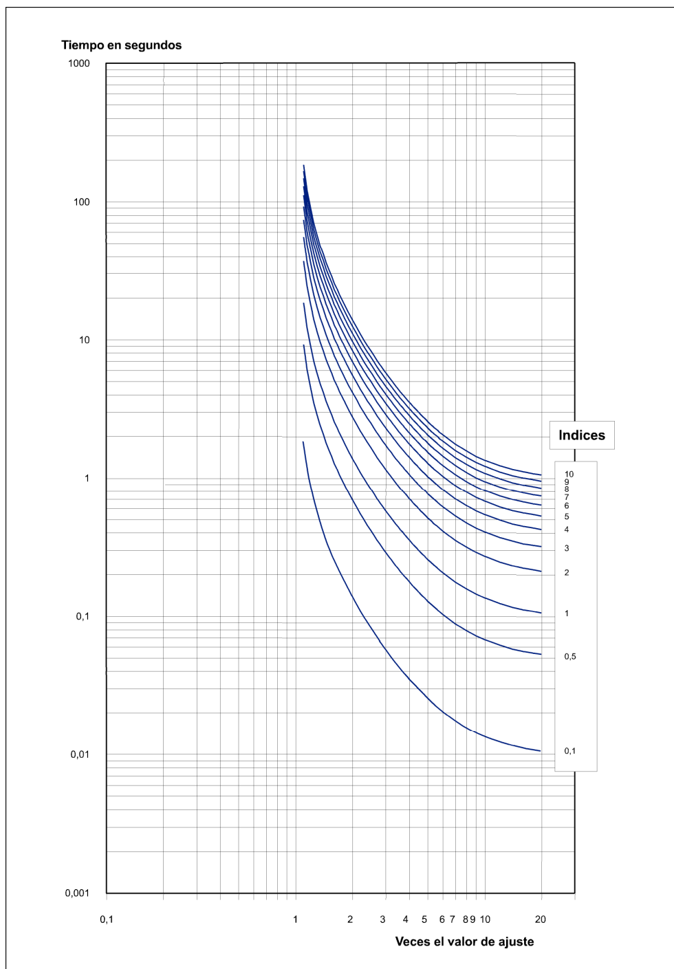
Figura 3.1.14: Característica MUY INVERSA (U.S.)
