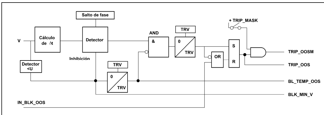
Figura 3.12.4: Diagrama de bloques de la unidad de salto de vector
