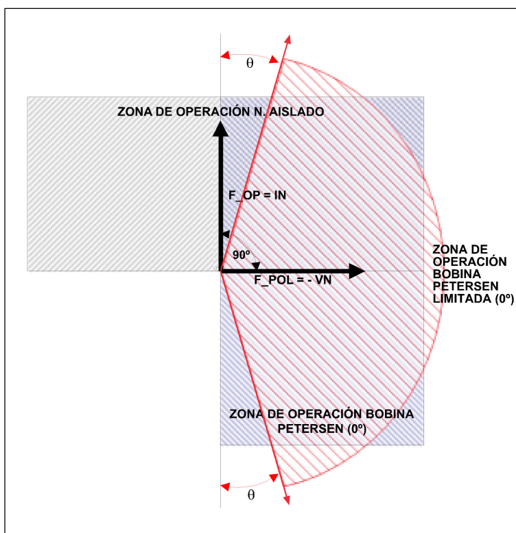
Figura 3.2.21: Diagrama vectorial de la característica de la unidad direccional de neutro aislado y de neutro compensado (bobina Petersen).
