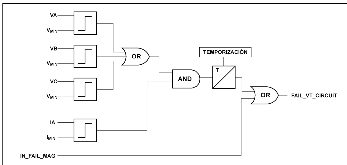
Figura 3.22.1: Diagrama de la unidad de detección de fallo en el circuito de tensión
