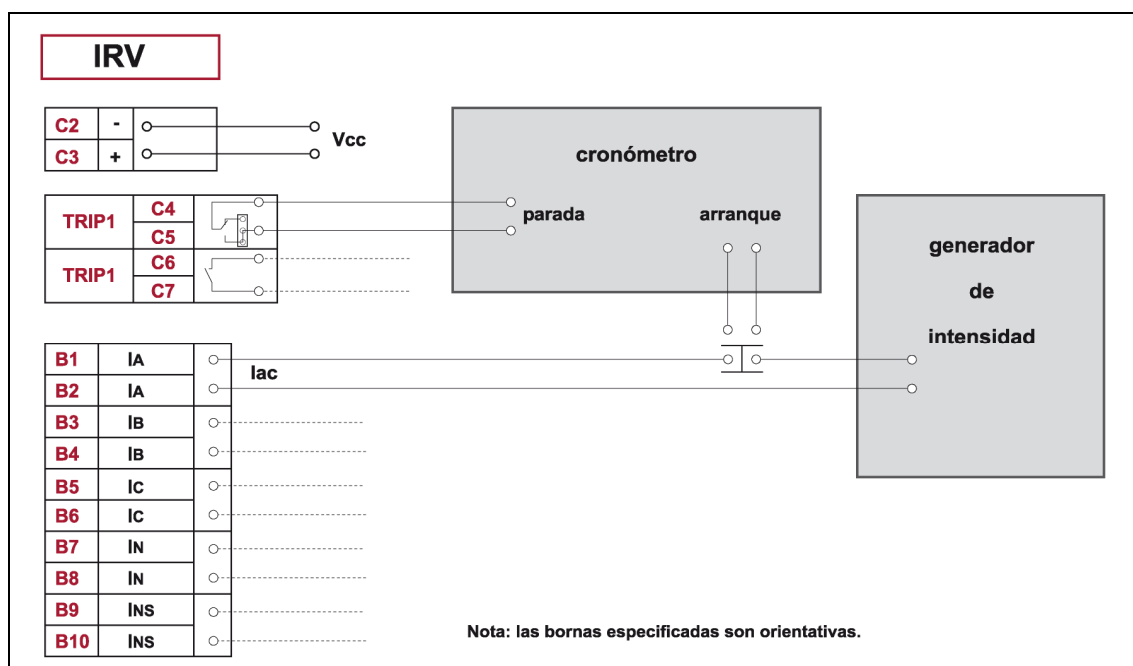
Figura 3.15.1: Esquema de conexión para el ensayo de medida de tiempos
