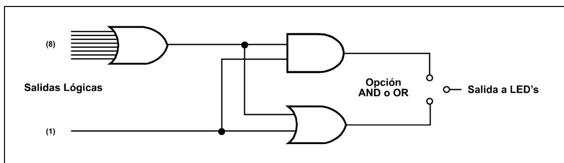
Figura 3.39.3: Diagrama de bloques de la celda lógica asociada a cada una de las salidas que actúan sobre los LEDs
