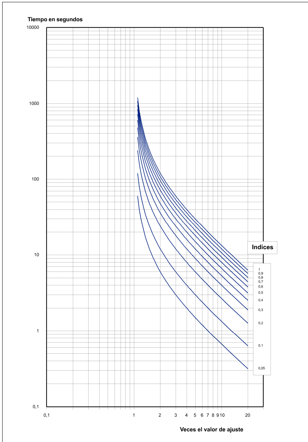
Figura 3.1.7: Característica TIEMPO-LARGO INVERSA (IEC)
