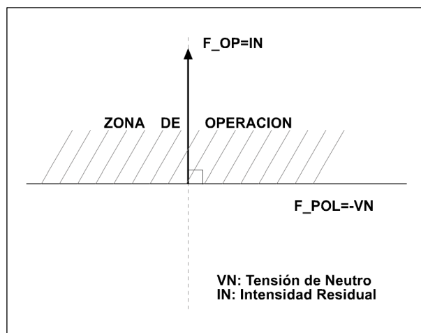
Figura 3.2.19: Diagrama vectorial de la característica de la unidad direccional de neutro aislado.
