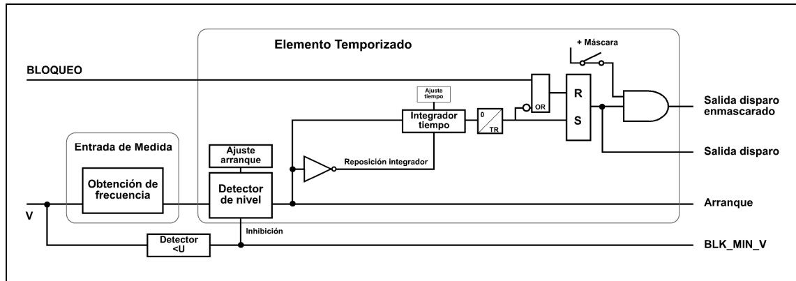
Figura 3.7.1: Diagrama de bloques de una unidad de frecuencia.
