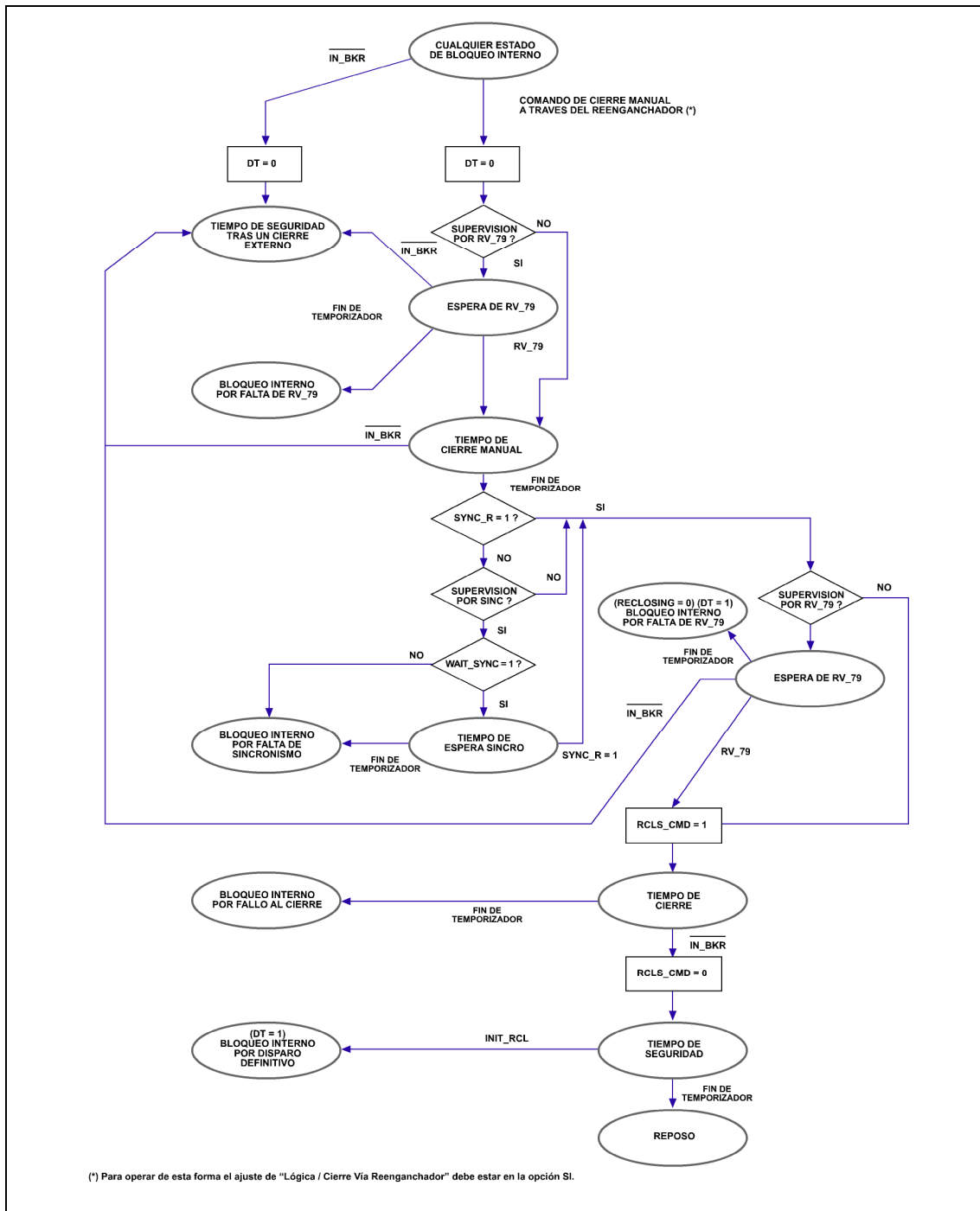
Figura 3.23.2: Diagrama de flujo del reenganchador (II)
