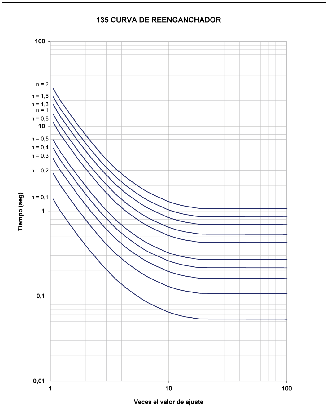
Figura 3.1.24: 135 curva de reenganchador
