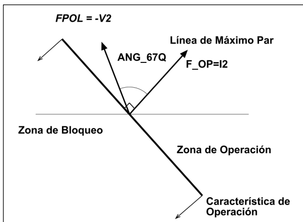
Figura 3.2.11: Diagrama vectorial de la unidad direccional de secuencia inversa.
