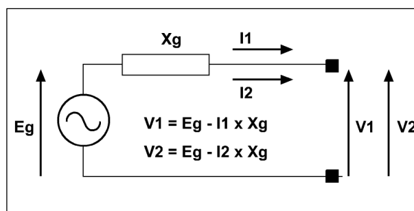
Figura 3.12.1: Circuito equivalente de un generador
