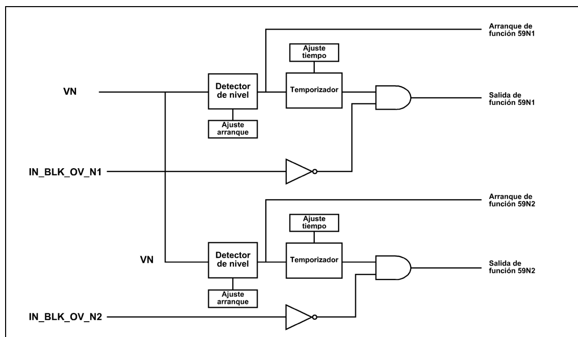
Figura 3.6.1: Diagrama de bloques de las unidades de sobretensión 59N1 y 59N2.
