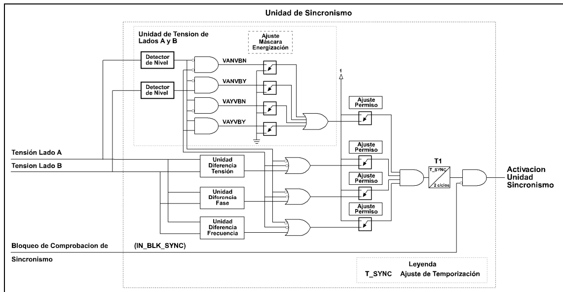
Figura 3.11.1: Diagrama de bloques de la unidad de sincronismo.
