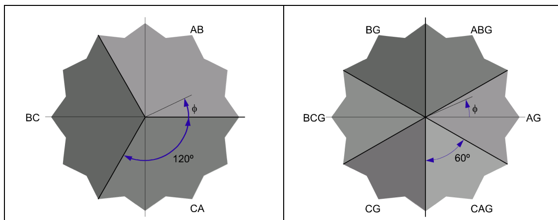
Figura 3.4.1: Diagrama de ángulo para faltas bifásicas
