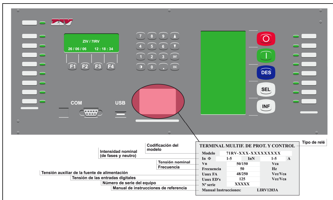
Figura 1.6.1: Placa de características (71RV)
