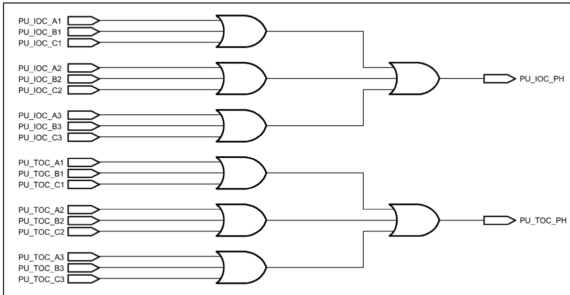
Figura 3.5.1: Lógica de activación de arranques de elementos de sobreintensidad de fase empleados por el detector de falta
