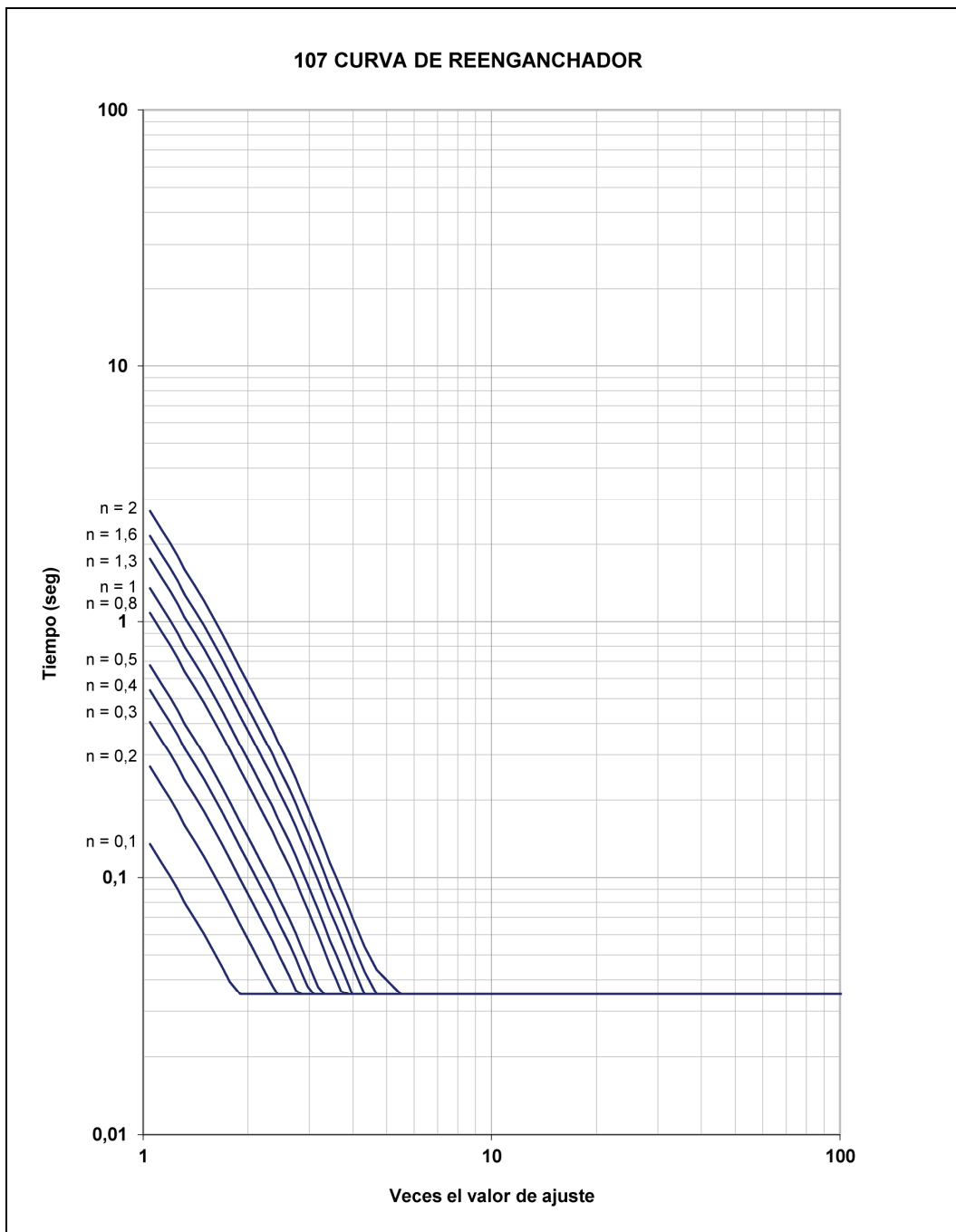
Figura 3.1.20: 107 curva de reenganchador
