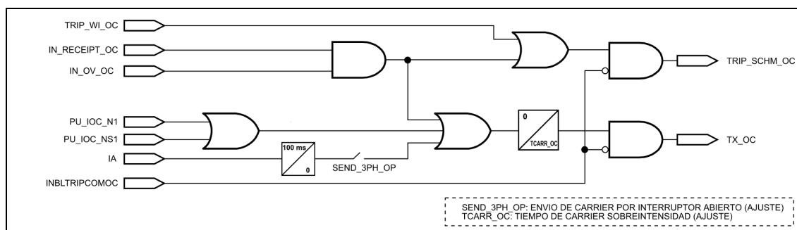
Figura 3.3.1: Diagrama de bloques del esquema de disparo por subcorte permisivo (IRV-D/G/H*****Y0)
