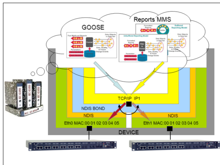
Figura 3.41.2: Configuración de los puertos de comunicaciones para el modelo con redundancia tipo Bonding.
