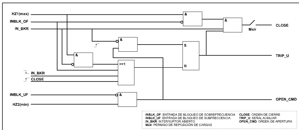
Figura 3.7.3: Diagrama lógico de deslastre de cargas para el tipo de deslastre subfrecuencia-sobrefrecuencia
