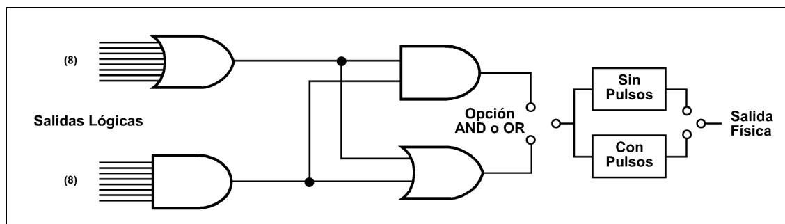
Figura 3.39.2: Diagrama de bloques de la celda lógica asociada a cada una de las salidas físicas
