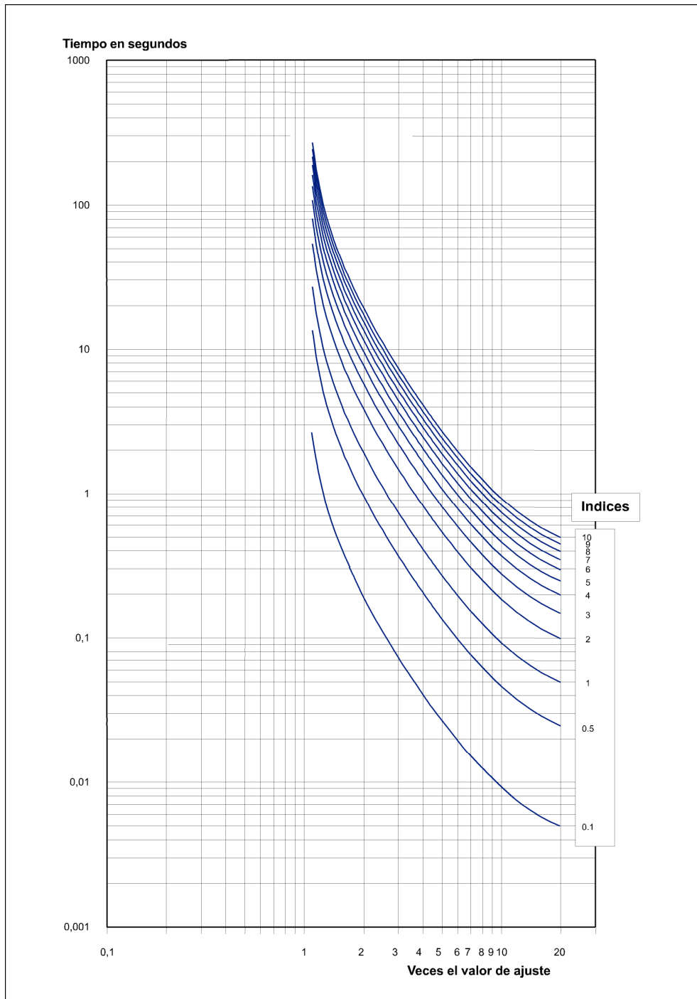
Figura 3.1.15: Característica EXTREMADAMENTE INVERSA (U.S.)
