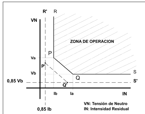
Figura 3.2.18: Diagrama de la característica de neutro aislado.
