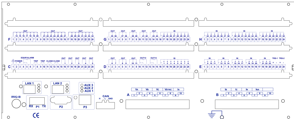
Figura 2.3.10: Trasera de un IRV de 4U de altura con bornas Phoenix
