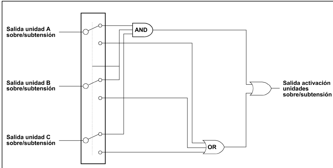
Figura 3.6.2: Diagrama de bloques de la operación AND / OR para las unidades de tensión.
