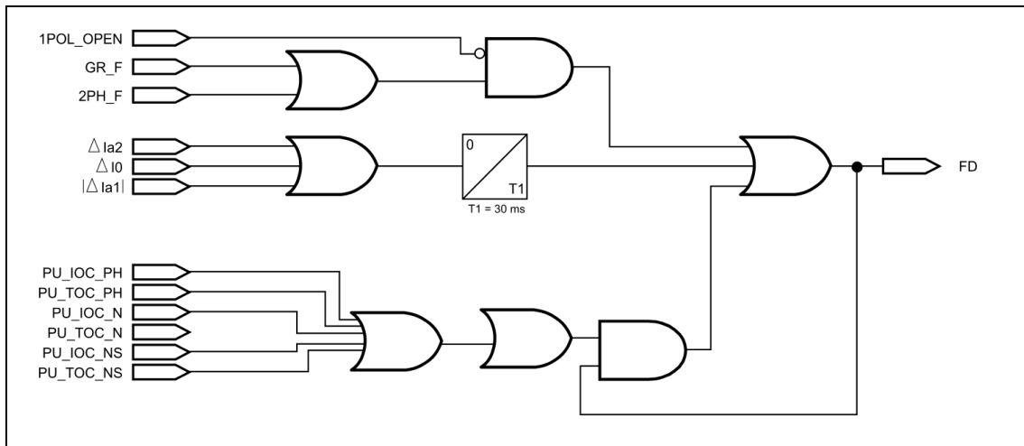
Figura 3.5.3: Diagrama de bloques del detector de falta
