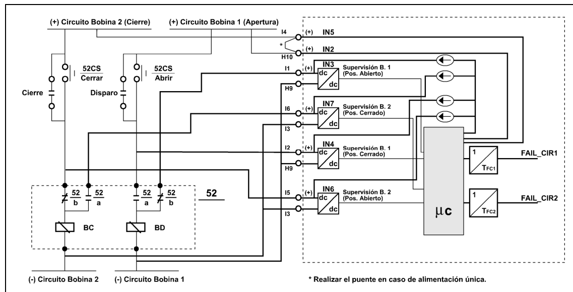
Figura 3.28.2: Diagrama de bloques y aplicación de las funciones de supervisión de circuitos de maniobra (II)
