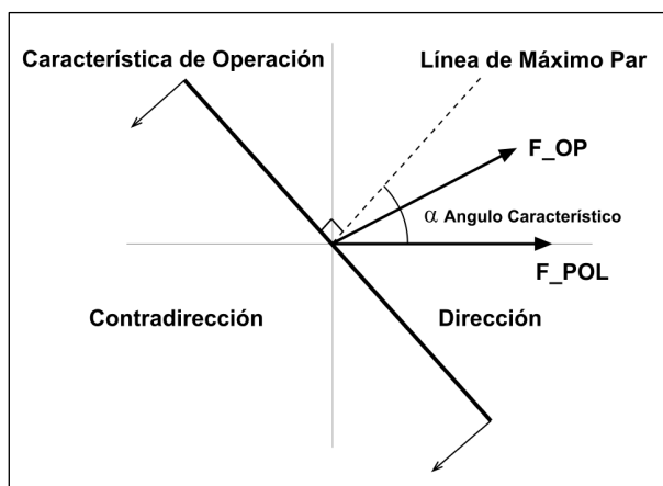
Figura 3.2.1: Diagrama vectorial de la unidad direccional de fase
