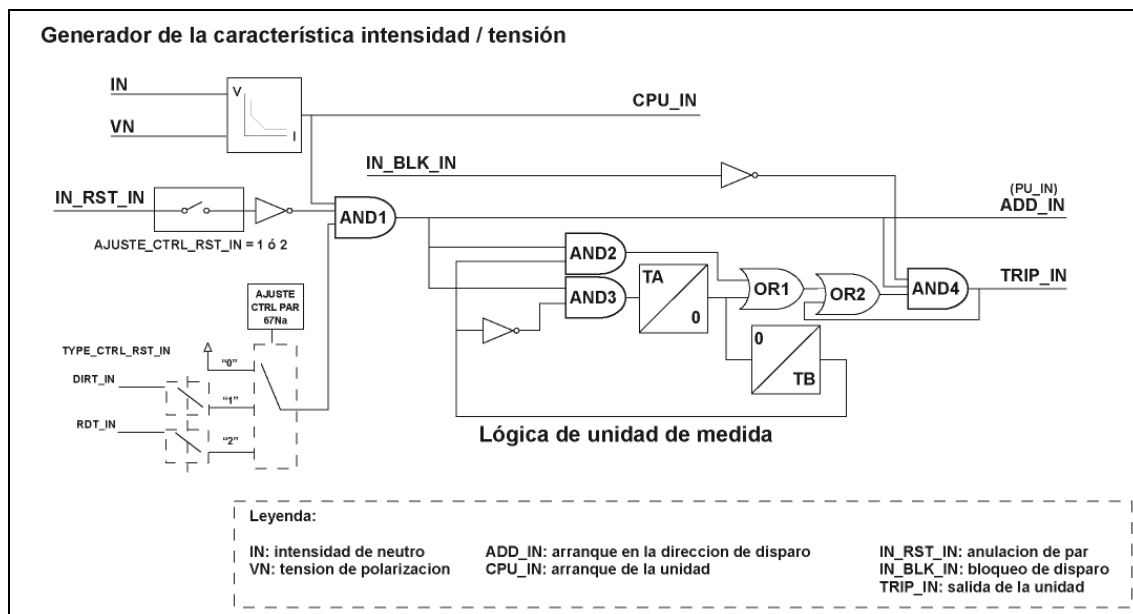
Figura 3.2.20: Lógica de la unidad de protección de neutro aislado.
