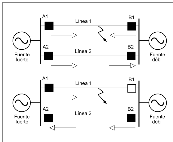
Figura 3.3.7: Fenómeno de inversión de intensidad
