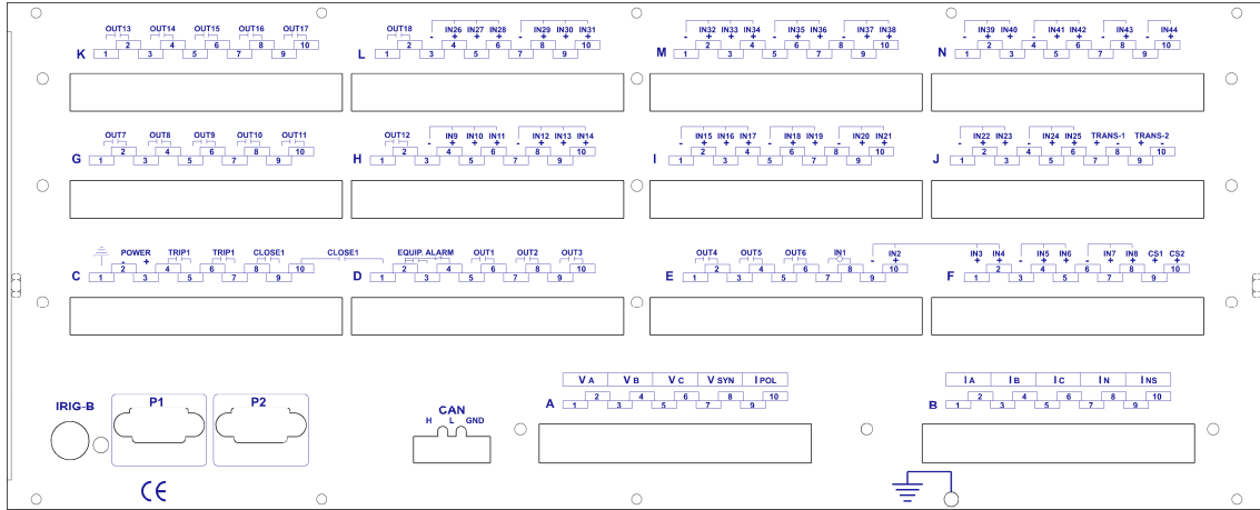
Figura 2.3.9: Trasera de un IRV de 4U de altura
