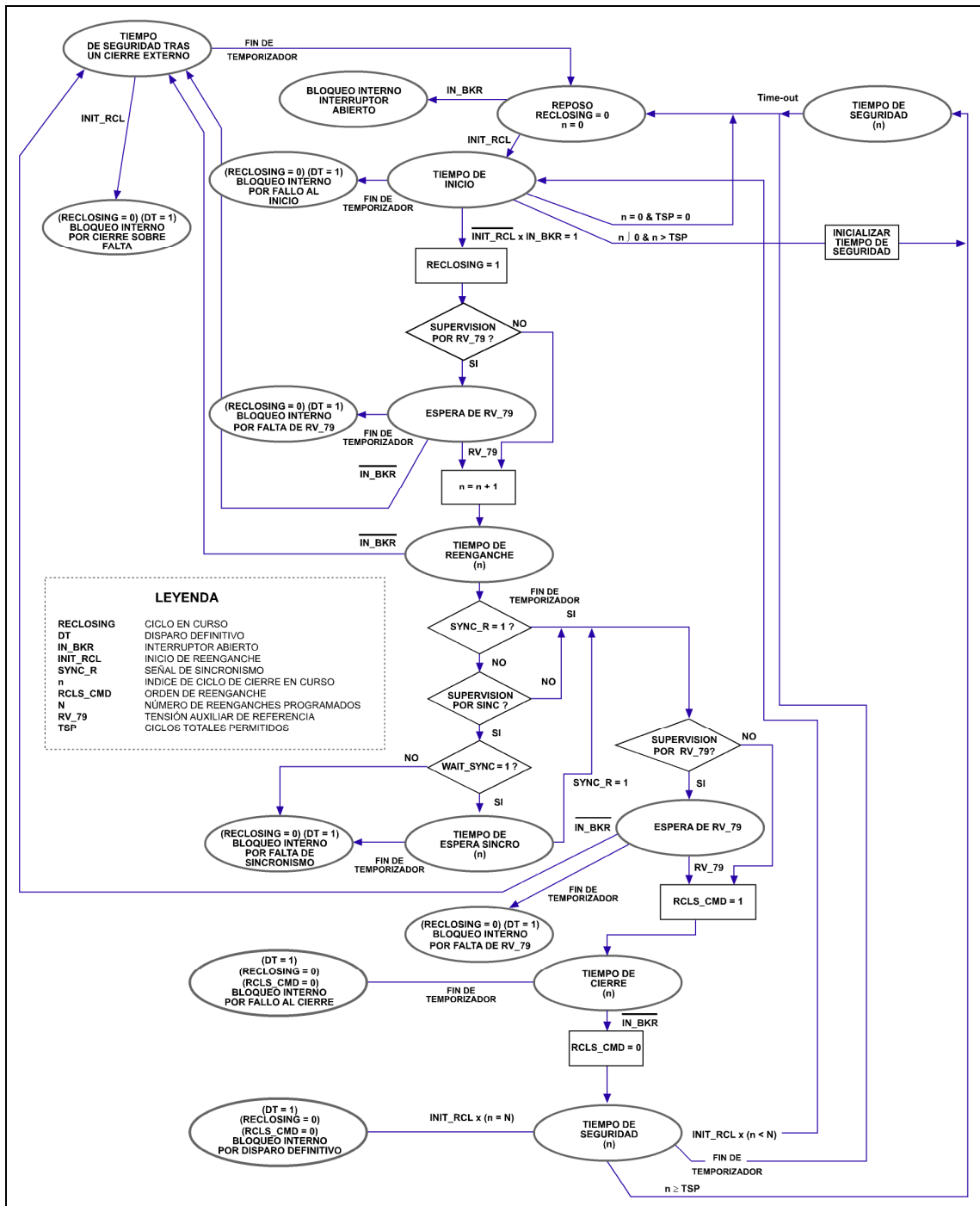
Figura 3.23.1: Diagrama de flujo del reenganchador (I)
