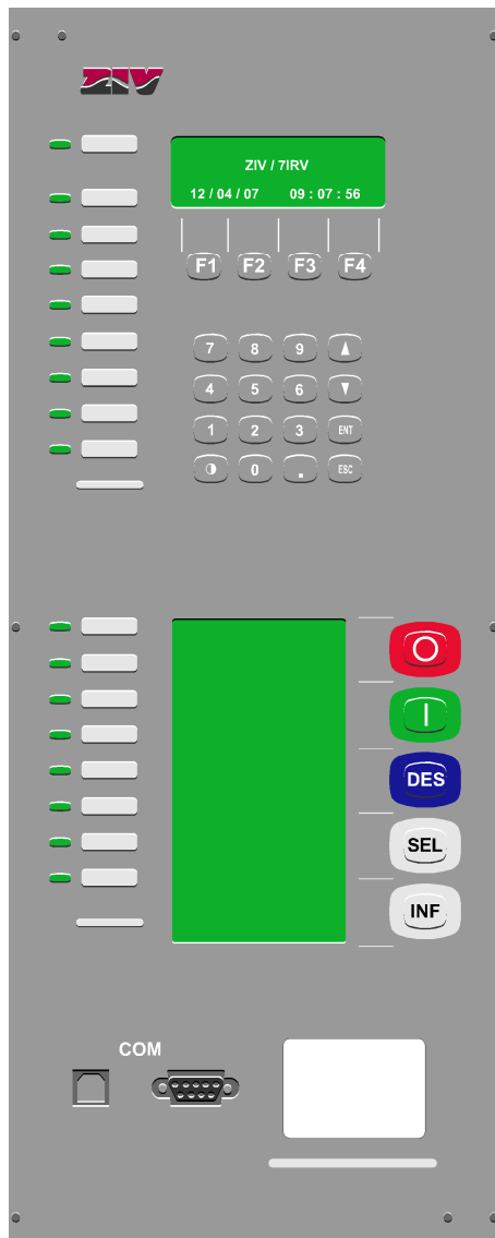
Figura 2.3.11: Frente de un 7IRV de 4U de altura en formato vertical
