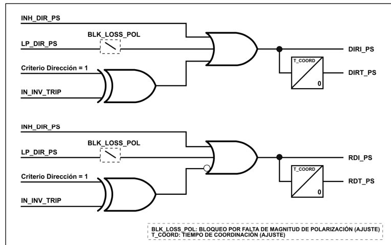
Figura 3.2.17: Diagrama de operación de la unidad direccional de secuencia directa.
