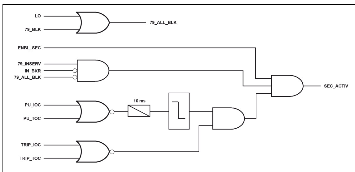
Figura 3.23.5: Lógica de coordinación de secuencia.
