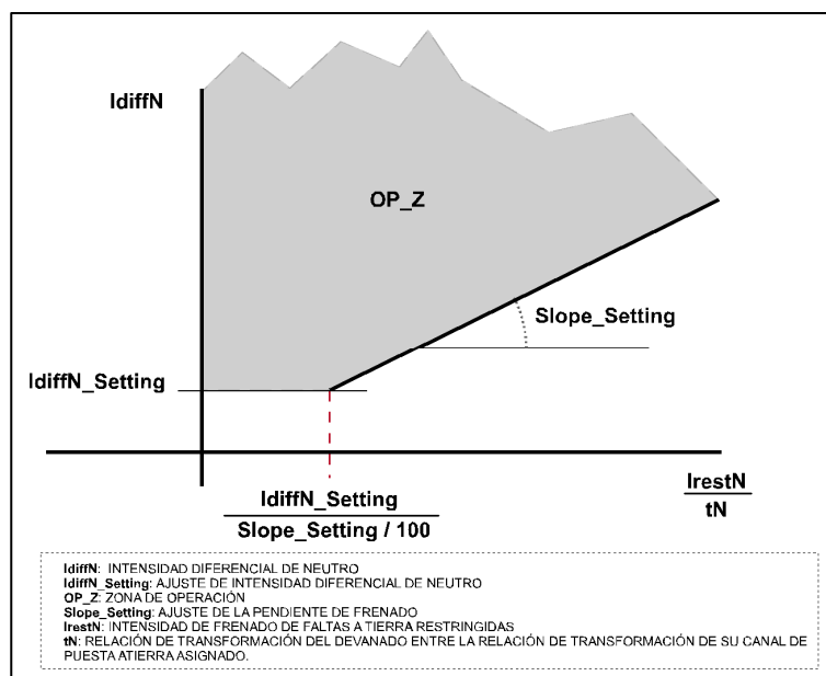
Figura 3.18.1: Característica de operación de la unidad de faltas a tierra restringidas.
