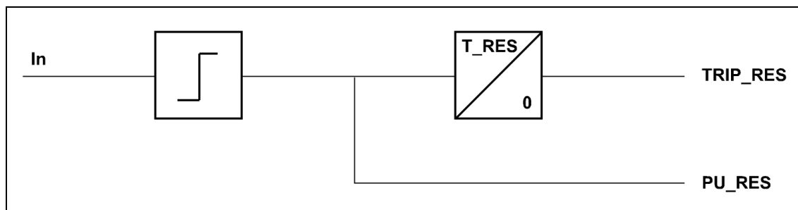
Figura 3.10.1: Diagrama de bloques de la unidad de detección de corriente residual
