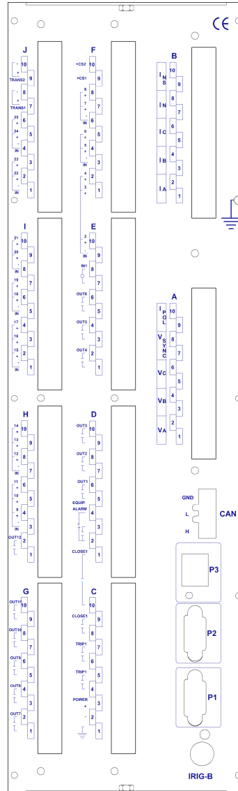
Figura 2.3.6: Trasera de un 3IRV
