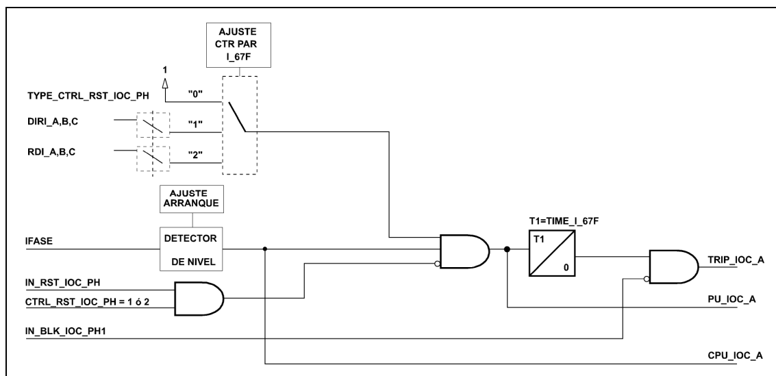
Figura 3.1.25: Diagrama de bloques de una unidad de sobreintensidad instantánea de fases
