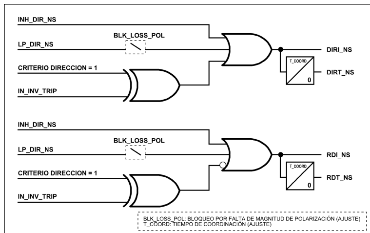
Figura 3.2.14: Diagrama de operación de la unidad direccional de secuencia inversa.
