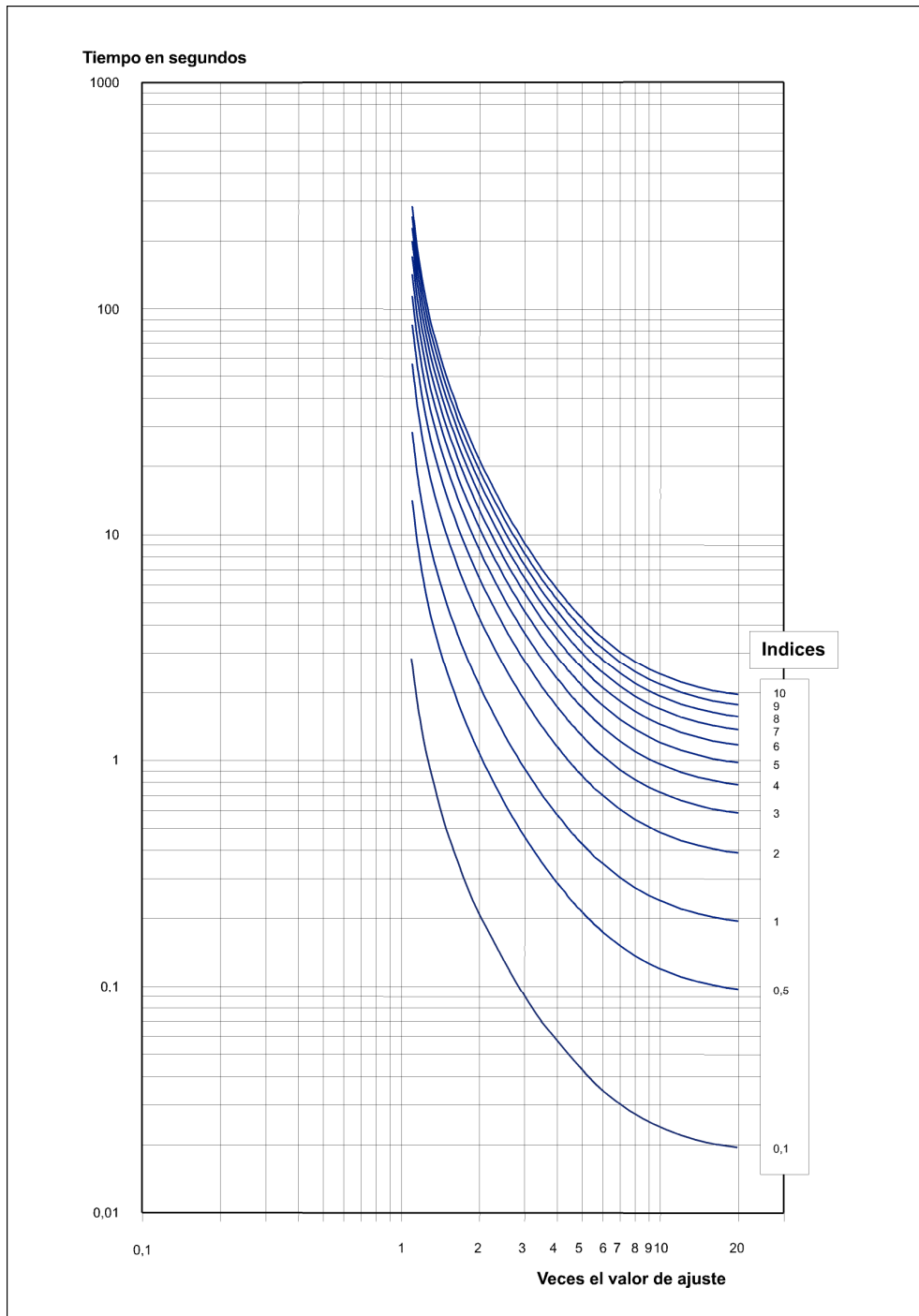
Figura 3.1.13: Característica INVERSA (U.S.)
