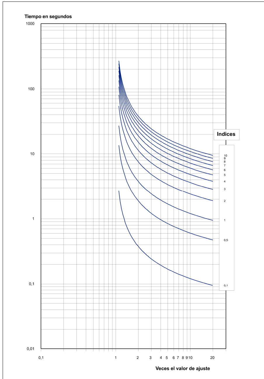
Figura 3.1.9: Característica MODERADAMENTE INVERSA (IEEE)
