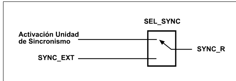
Figura 3.23.4: Señal de sincronismo
