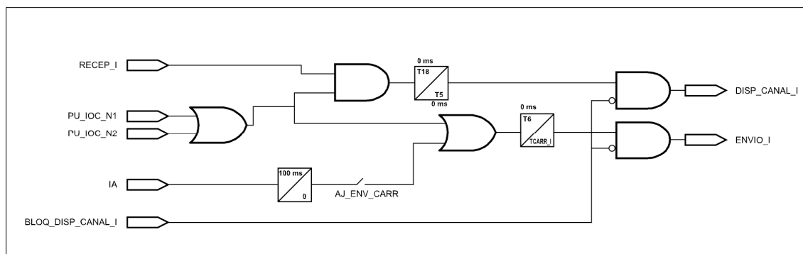
Figura 3.3.3: Diagrama de bloques del esquema de disparo por sobrealcance permisivo para sobreintensidad
