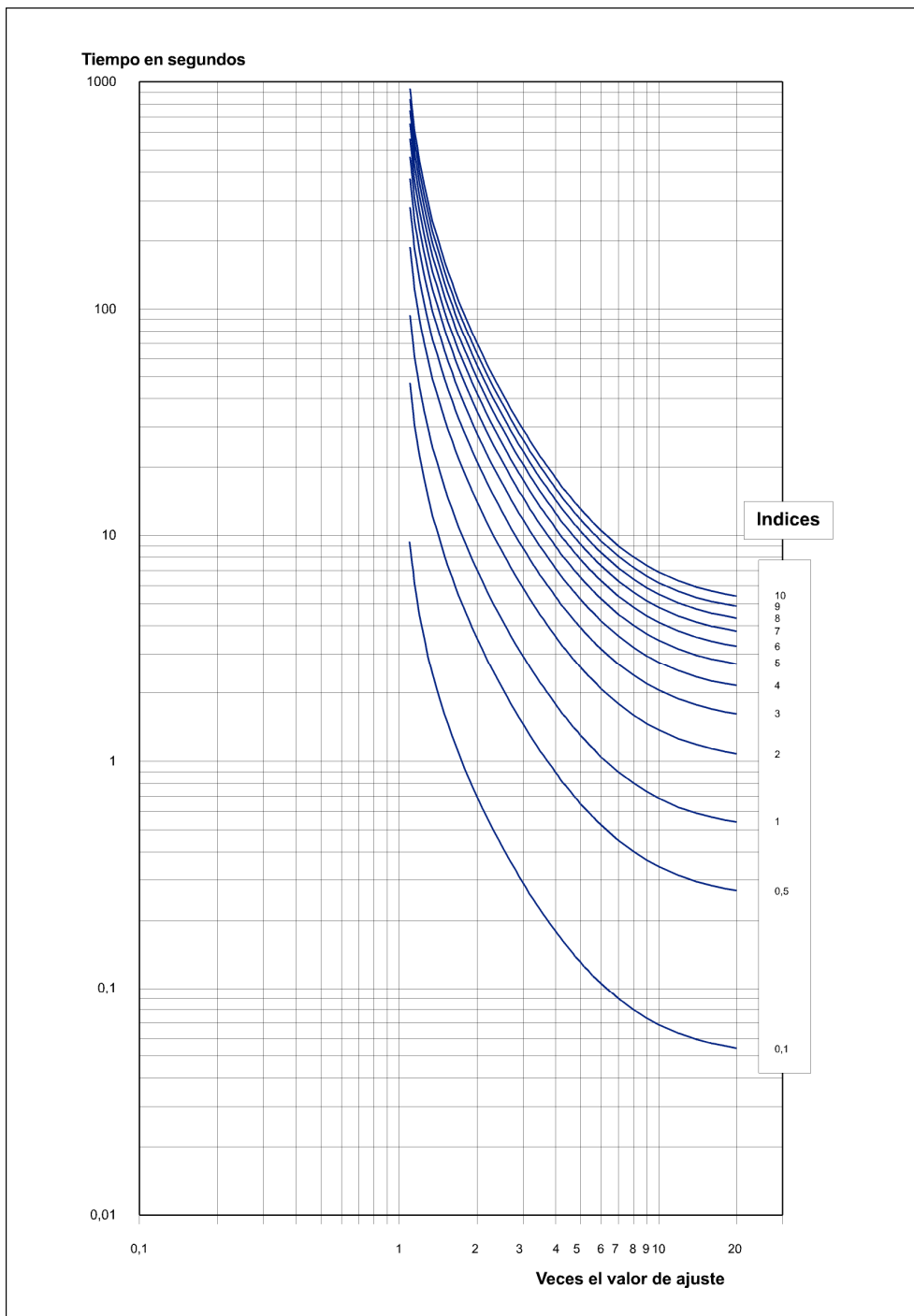
Figura 3.1.10: Característica MUY INVERSA (IEEE)
