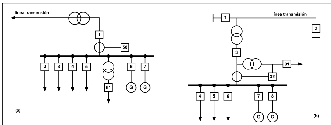
Figura 3.7.4: Sistema de deslastre de cargas en una planta industrial.
