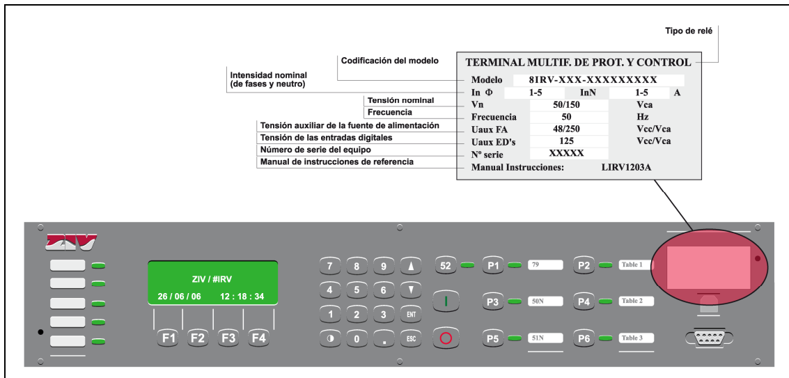
Figura 1.6.2: Placa de características (8IRV)
