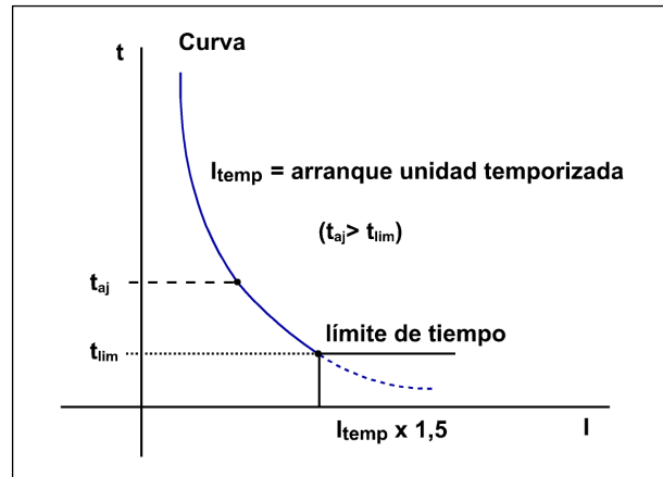
Figura 3.1.3: Diagrama de una curva con límite de tiempo para el caso de tiempo fijo mayor que el tiempo de curva (en arranque x 1,5)
