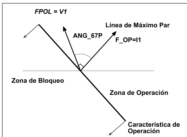
Figura 3.2.16: Diagrama vectorial de la unidad direccional de secuencia directa.
