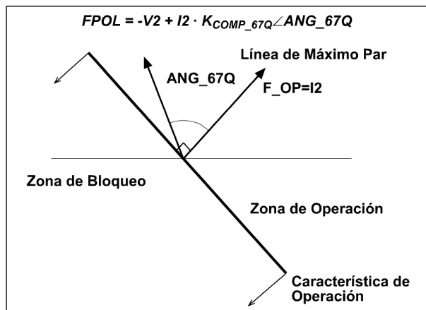
Figura 3.2.15: Diagrama vectorial de la unidad direccional de secuencia inversa de los modelos IRV-D*****Y0 e IRV-J.
