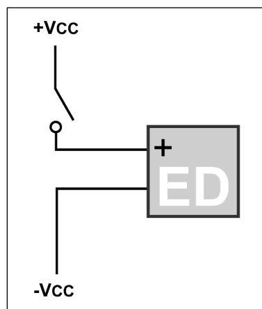
Figura 3.39.4: Ensayo de las entradas digitales
