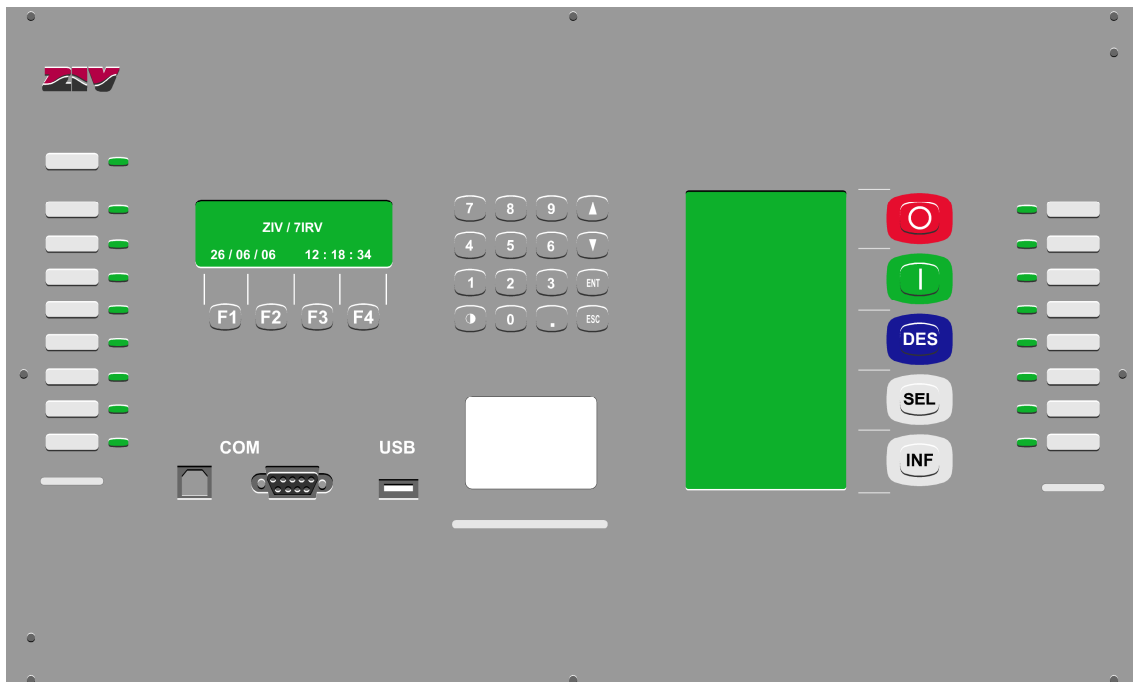
Figura 2.3.14: Frente de un 7IRV de 6U de altura
