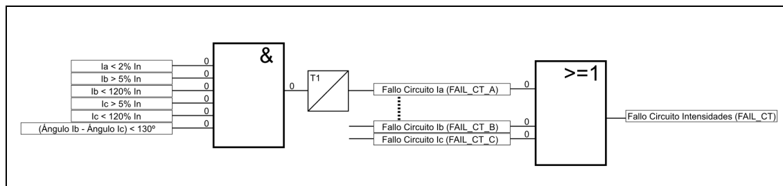
Figura 3.21.1: Algoritmo de supervisión para la medida de intensidad de la fase A
