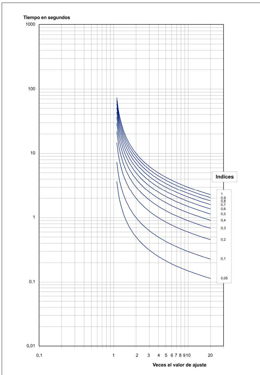
Figura 3.1.4: Característica INVERSA (IEC)
