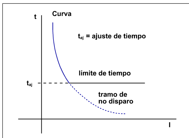
Figura 3.1.2: Diagrama de una curva con límite de tiempo para una unidad de sobreintensidad temporizada
