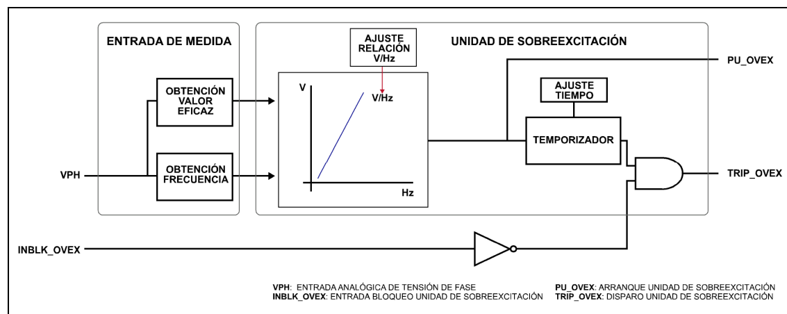
Figura 3.19.1: Diagrama de bloques de la unidad de sobreexcitación.
