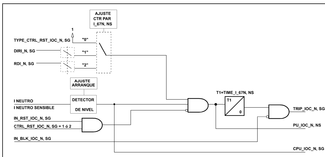
Figura 3.1.26: Diagrama de bloques de una unidad de sobreintensidad instantánea de neutro y neutro sensible
