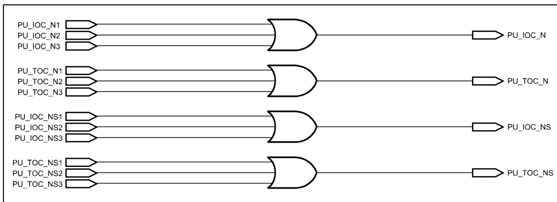
Figura 3.5.2: Lógica de activación de arranques de elementos de sobreintensidad de neutro y secuencia inversa empleados por el detector de falta
