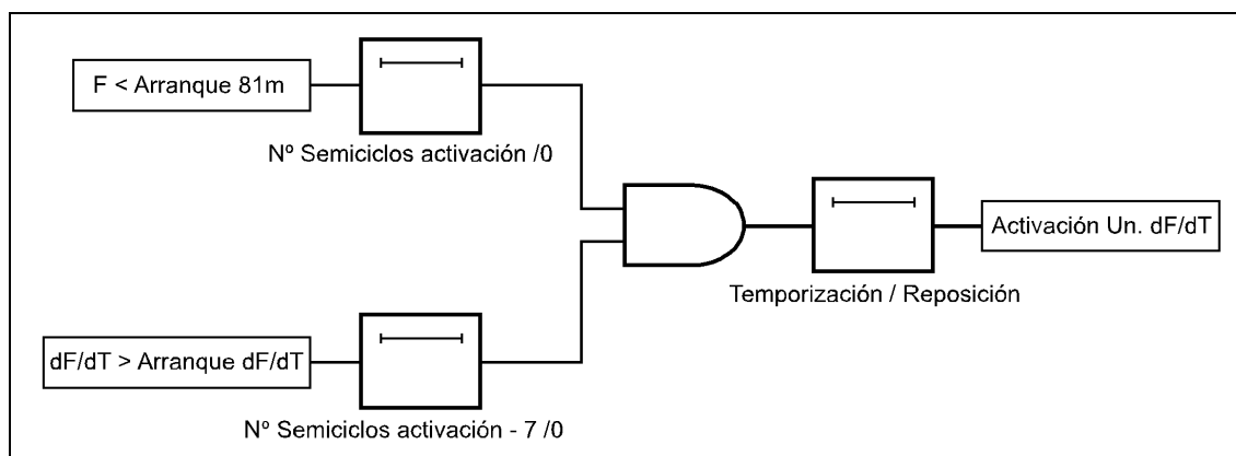
Figura 3.7.2: Lógica de una unidad de derivada de frecuencia
