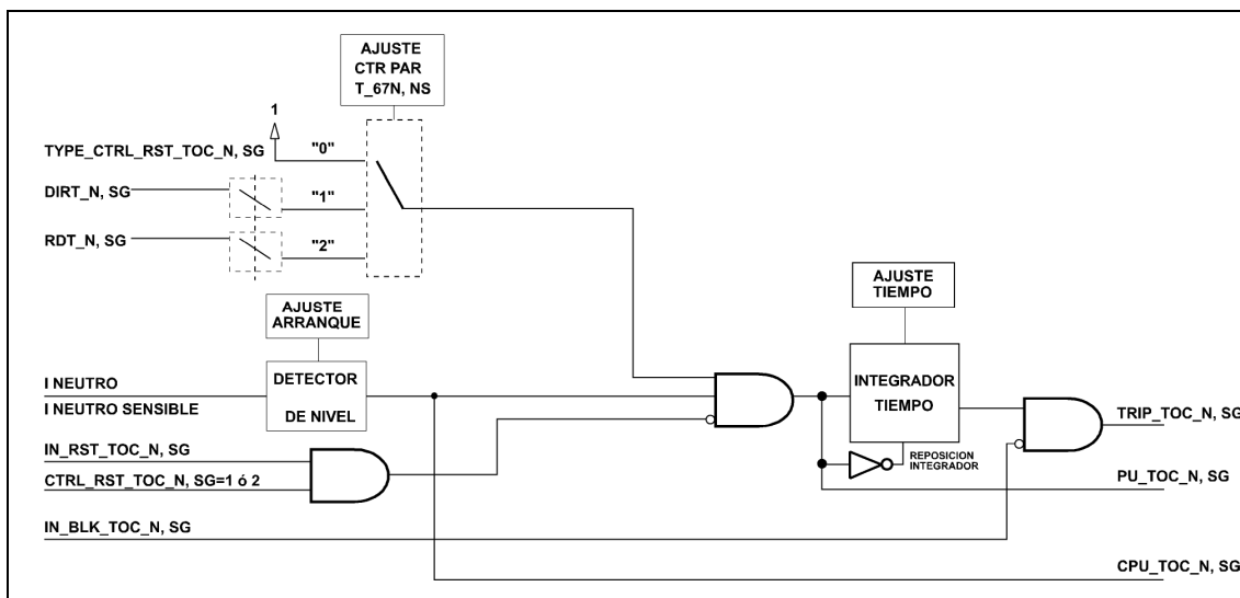
Figura 3.1.28: Diagrama de bloques de una unidad de sobrecorriente temporizada de neutro y neutro sensible
