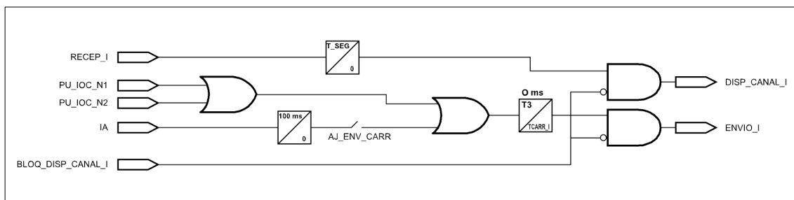
Figura 3.3.2: Diagrama de bloques del esquema de disparo transferido directo para sobreintensidad
