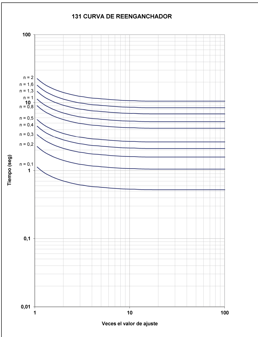
Figura 3.1.23: 131 curva de reenganchador
