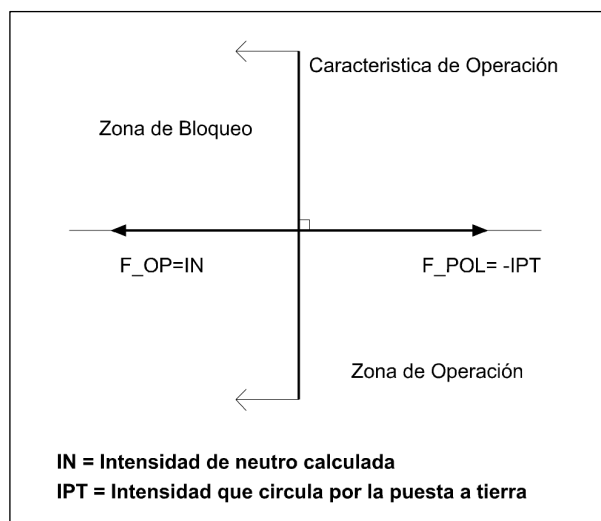
Figura 3.2.8: Diagrama vectorial de la unidad direccional de neutro (polarización por intensidad)
