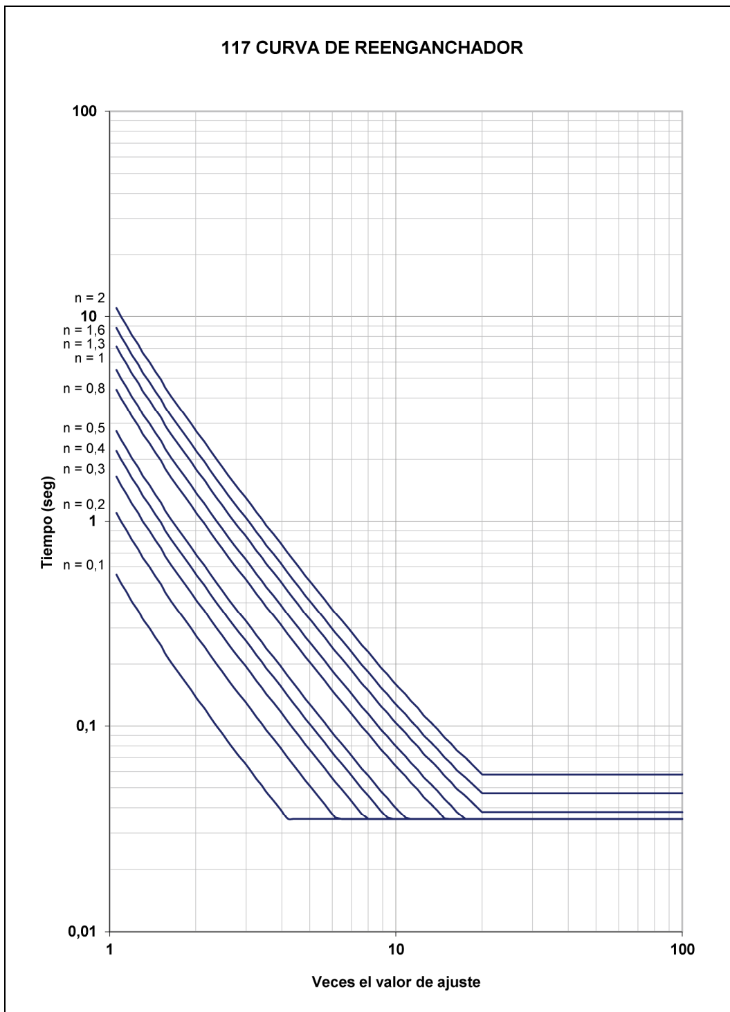
Figura 3.1.22: 117 curva de reenganchador
