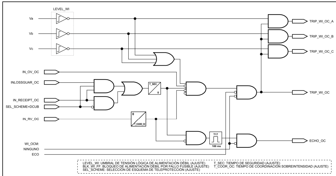
Figura 3.3.6: Diagrama de bloques de la lógica de alimentación débil (IRV-D/G/H****Y0 e IRV-J)
