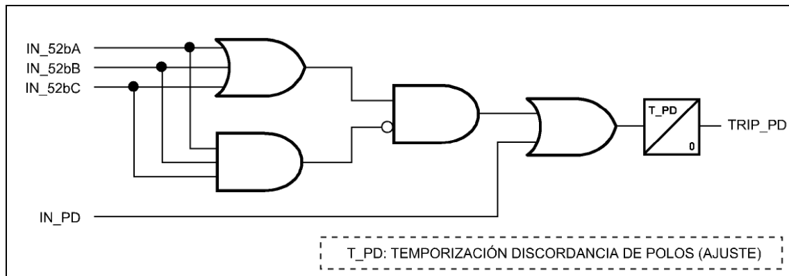
Figura 3.29.1: Diagrama del detector de discordancia de polos
