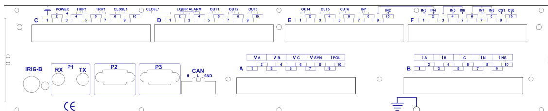
Figura 2.3.2: Trasera de un 8IRV de 2U de altura
