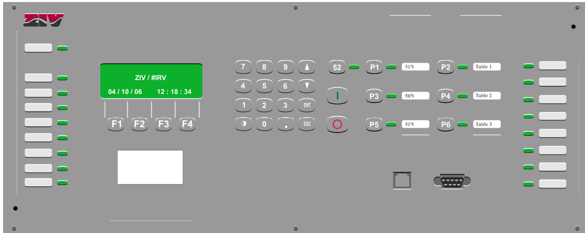
Figura 2.3.7: Frente de un 8IRV de 4U de altura
